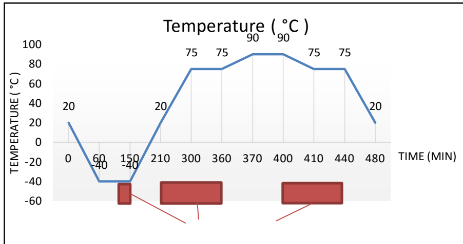
Kuva 12. Yhden jakson lämpötilaprofiili sekä toiminnallisuuden testauksen ajankohdat
