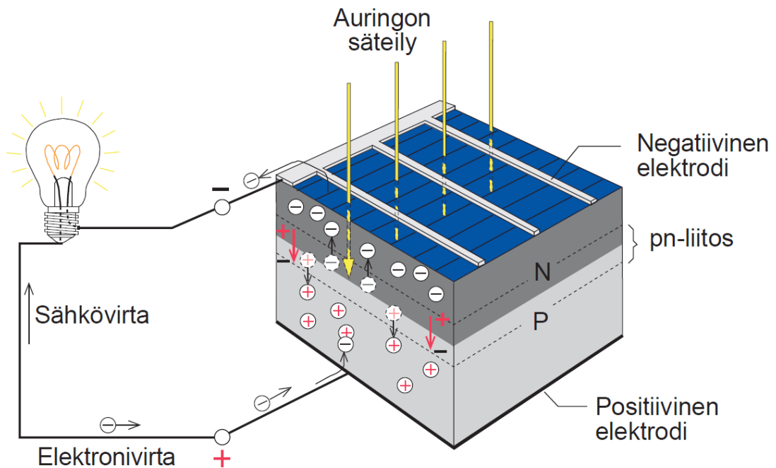
KUVA 12. Aurinkokennon rakenne ja toiminta (Paavola, 2014)
