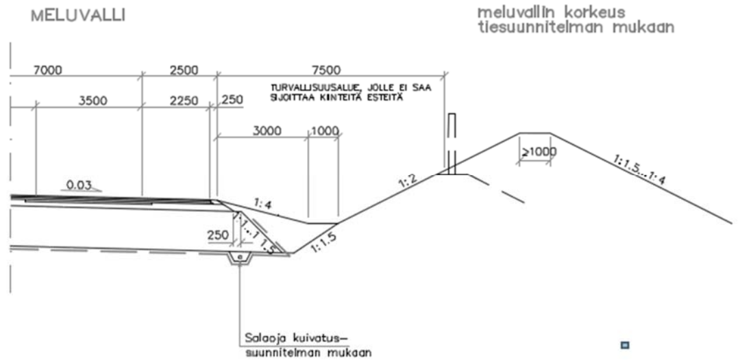
Kuva 5. Tien rakenteellinen tyypipoikkileikkaus. [5.]
