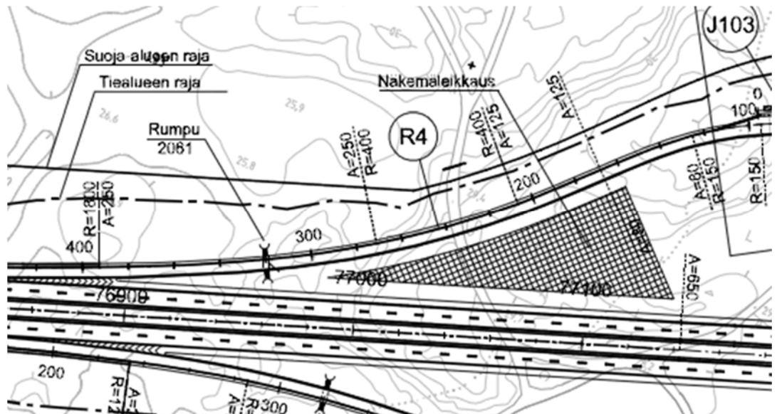
Kuva 2. Tie rakennussuunnitelman väylägeometria ja aluerajat rakennussuunnitelmakartassa. [5.]
