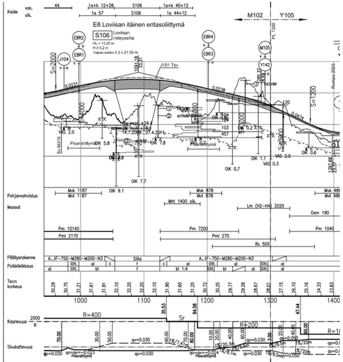
Kuva 6. Tien rakennussuunnitelman pituusleikkaus. [5.]
