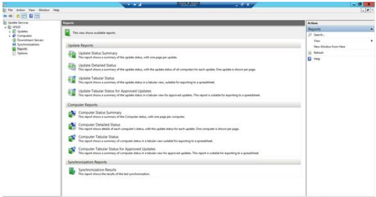
Kuva 9. Reports -valikko.
