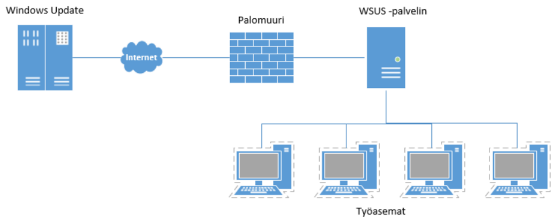
Kuva 3. Projektityöympäristön toiminta.
