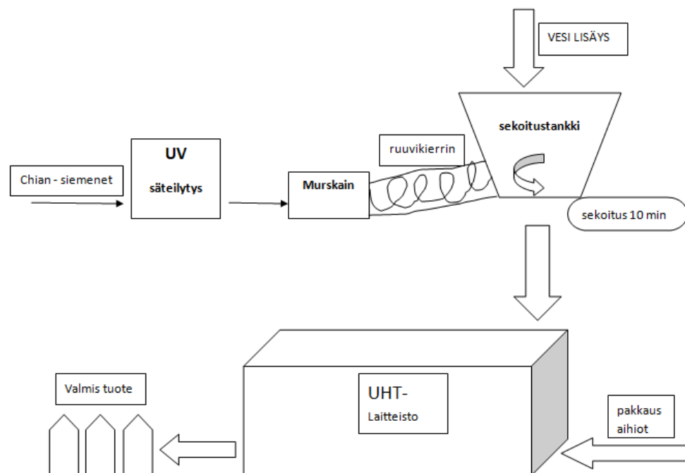
Kuva 14. Prosessin vuokaavio.
