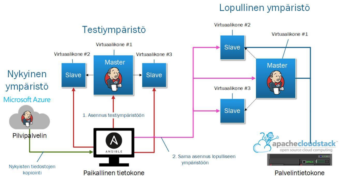
Kuva 3. Suunniteltu prosessikokonaisuus
