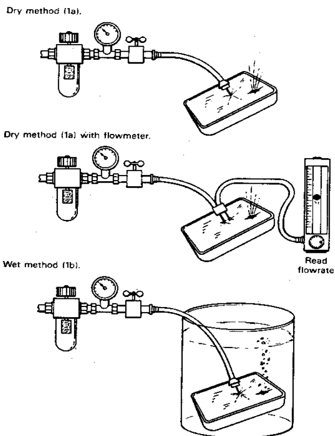
Kuva 16. Painetestin suoritusmekanismia [28].
