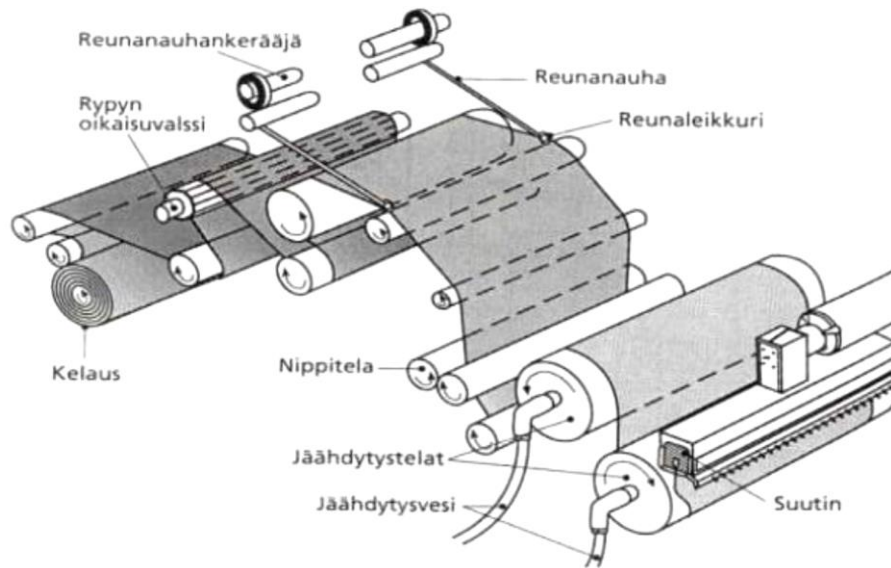
Kuva 9. Tasokalvokone [17, s. 108].
