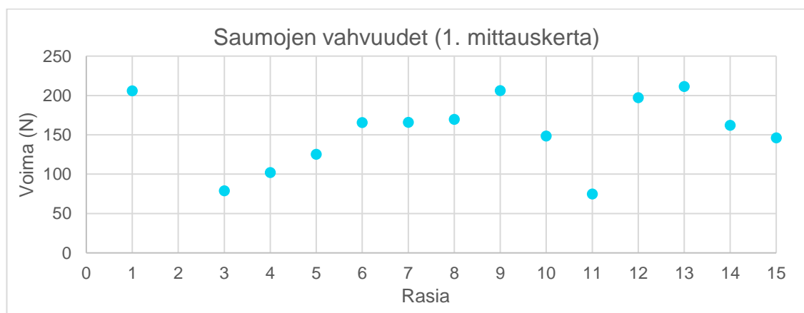
Kuva 22. Rasioiden saumojen vahvuudet ensimmäisellä mittauskerralla
