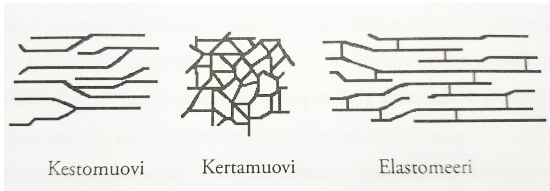
Kuva 1. Kestomuovin, kertamuovin ja elastomeerin polymeerirakenteet [7, s. 28].
