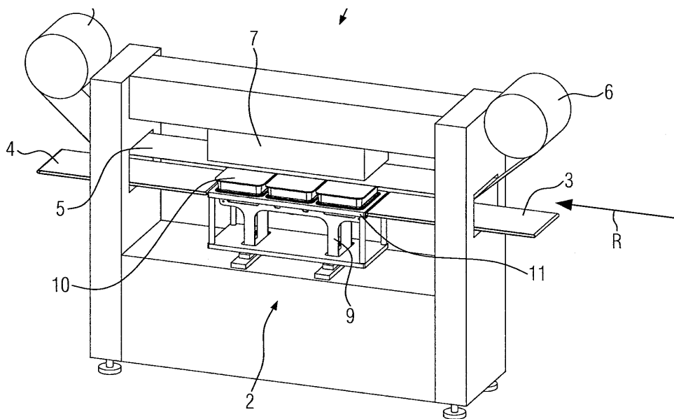
Kuva 18. Automaattinen alustapakkaus kone [37].
