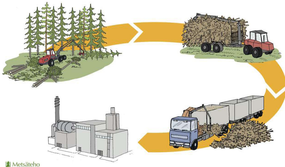
KUVIO 10. Hakkuutähteen tienvarsihaketuksen tuotantoketju, integroidulla hakkuri-hakeautolla (Metla 2008).
