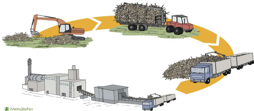
KUVIO 12. Kantomurskeen tuotantoketju, käyttöpaikkamurskaus menetelmällä (Metla 2008).
