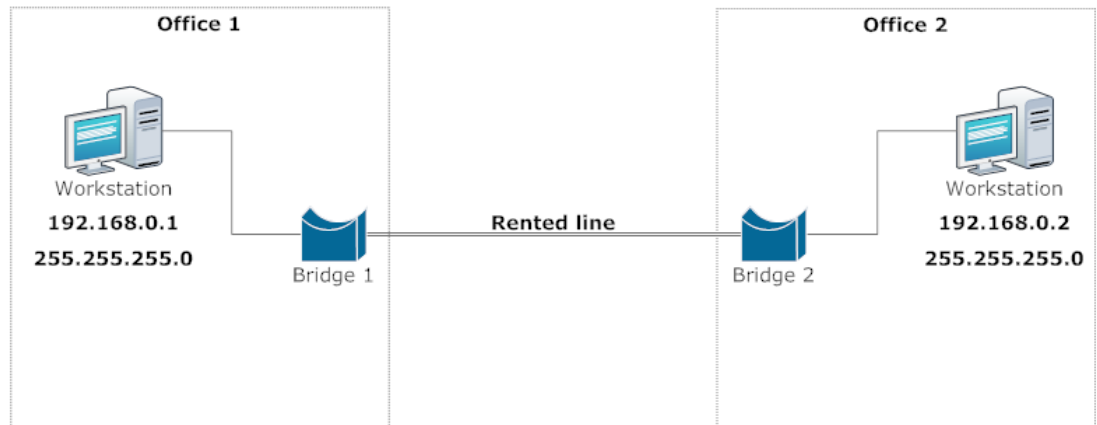
KUVA 5. Etäsilta
