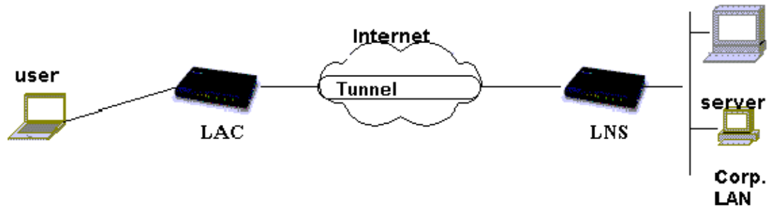
KUVA 10. L2TP tunneli [18]
