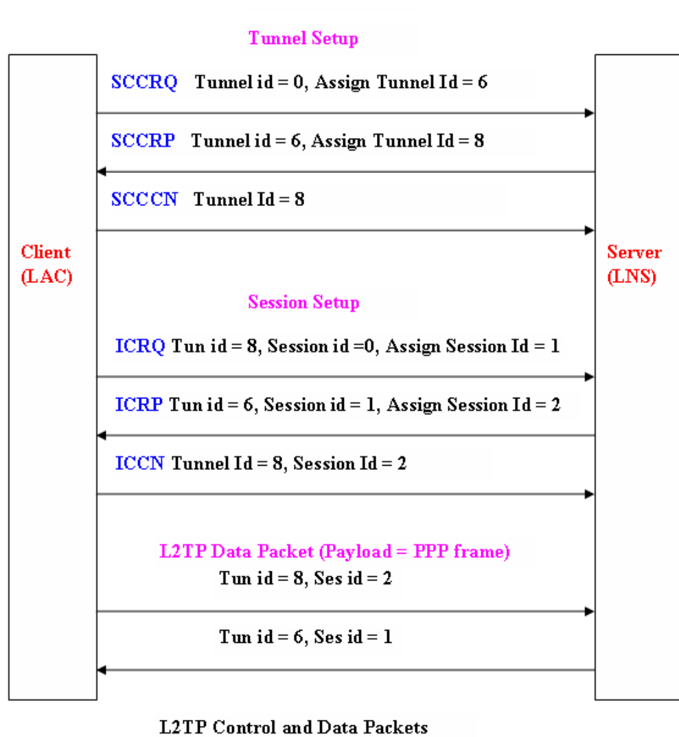
KUVA 11. L2TP yhteyden muodostaminen [17]
