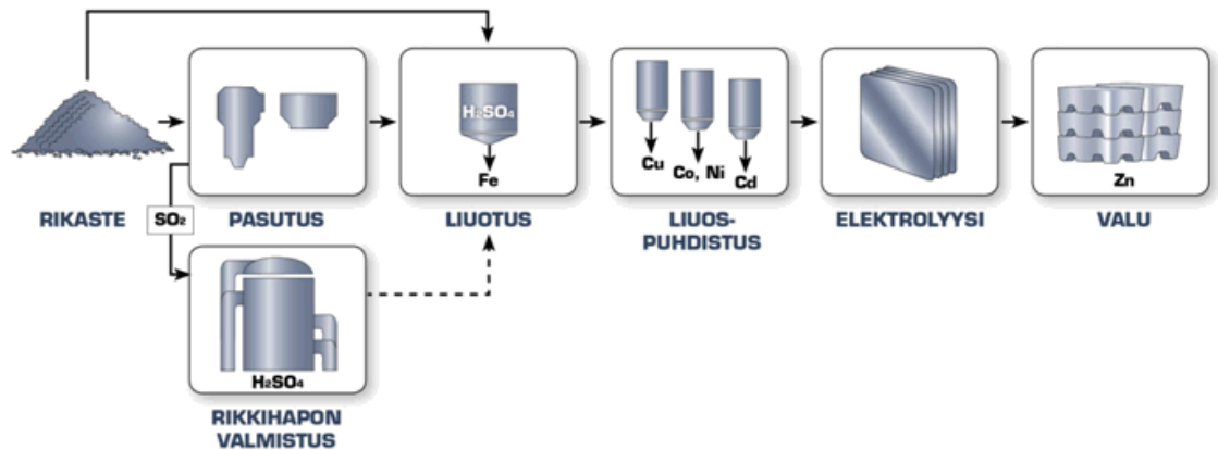
KUVIO 1. Sinkin tuotantoprosessi (New Boliden d 2011.)
