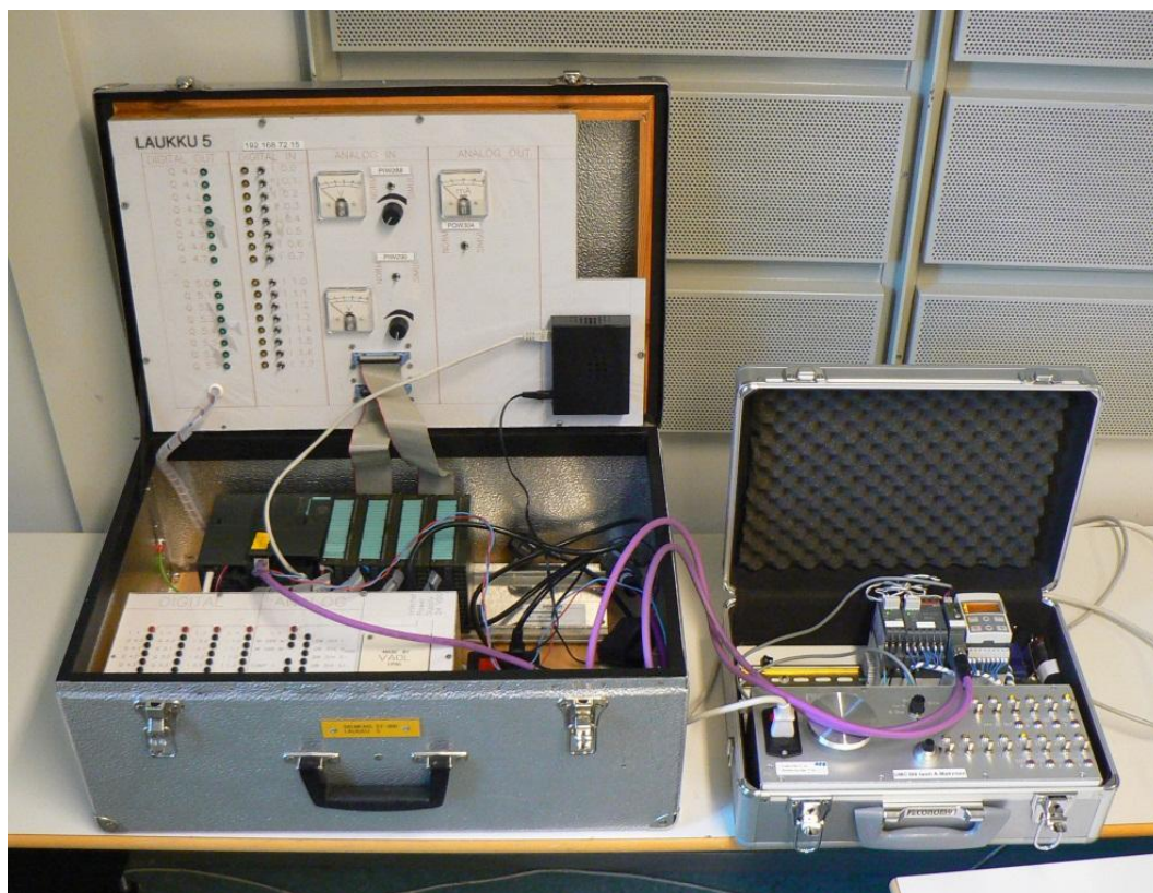
Kuvio 29. S7-kokoonpano ja UMC100-demolaitteisto. /9./
