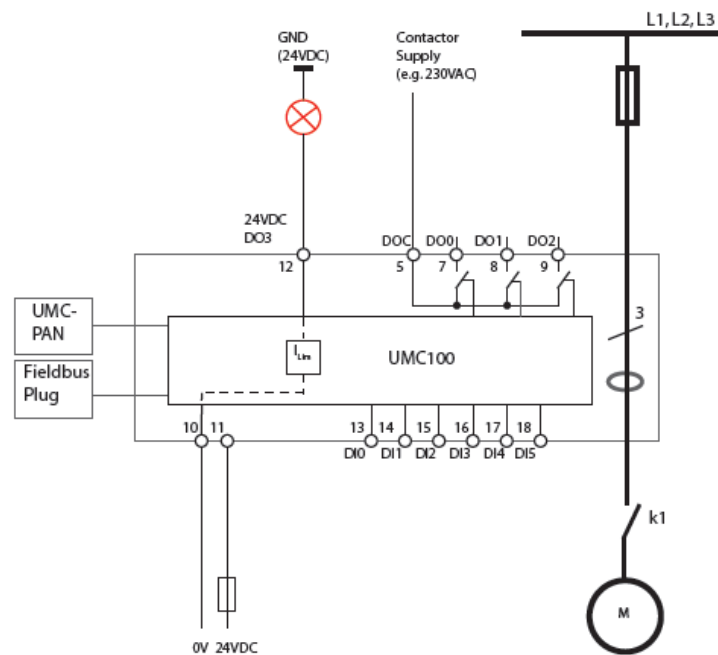
Kuvio 15. Transparent-ohjaustoiminnojen piirikaavion esimerkki. /16./
