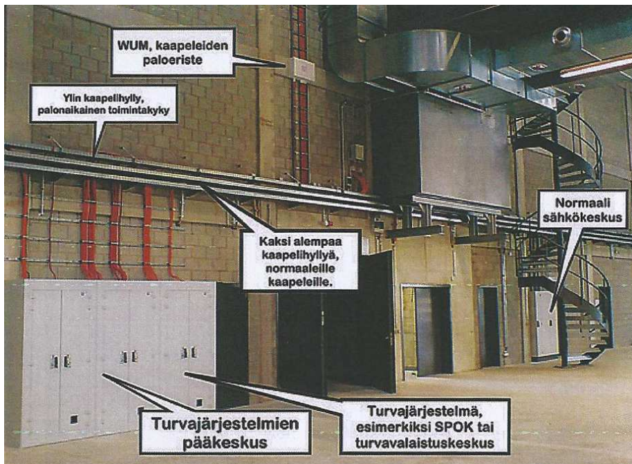
Kuva 13. Turvajärjestelmien keskukset sijoitettuna erilleen normaalin syötön keskukselta [2].
