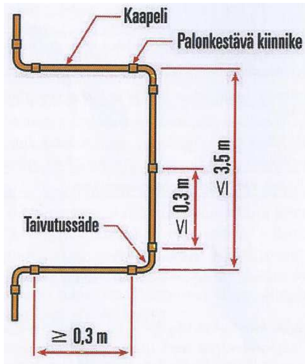
Kuva 9. Vektorituksen pienentäminen pystysuorassa kaapeliasennuksessa [2].
