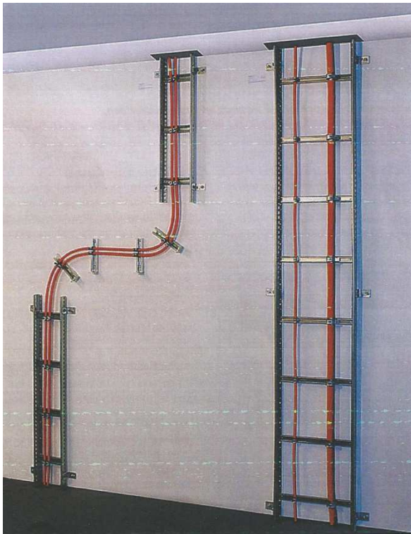
Kuva 4. Pystysuorat kaapeli-asennukset oikein toteutettuina [2].
