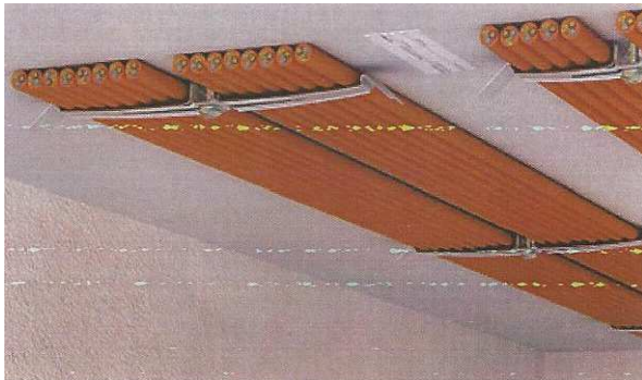
Kuva 11. Kaapelit asennettuina suoraan kattopintaan [2].
