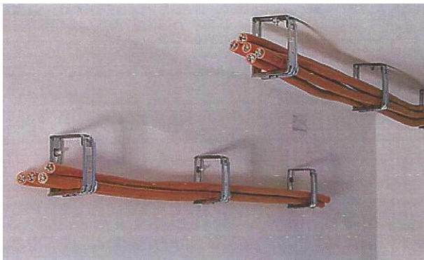
Kuva 12. Kaapeliniiput asennettuina seinä- ja kattopintaan [2].
