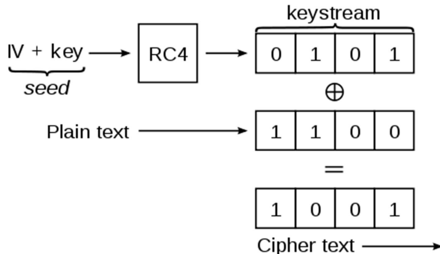
Kuva 4. WEP-suojausmenetelmä.
