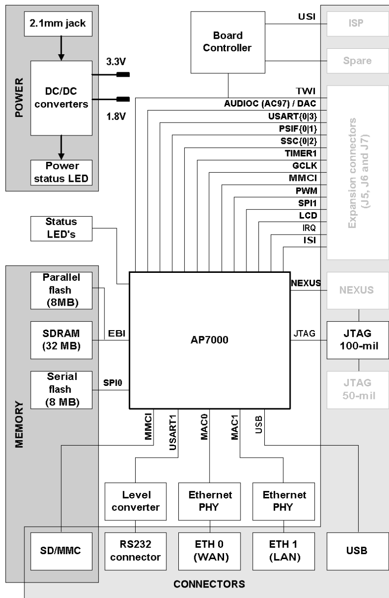
Kuva 2. NGW lohkokaaavio /5/
