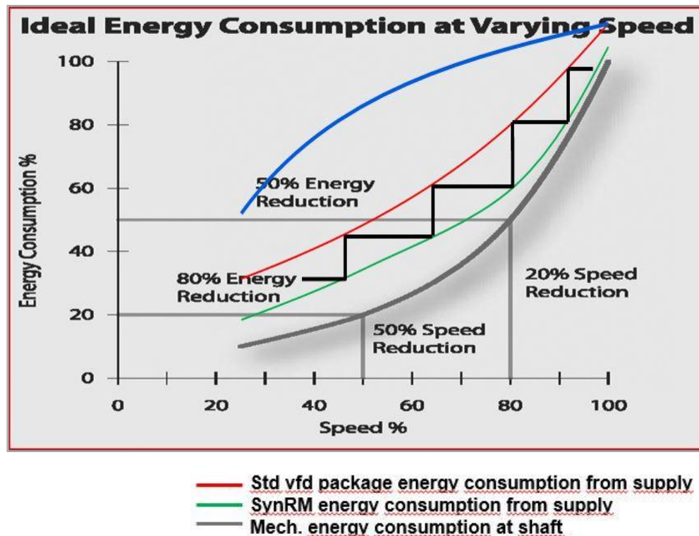
KUVA 14. Prosessin energiansäästö ja hyötysuhteen muutos
