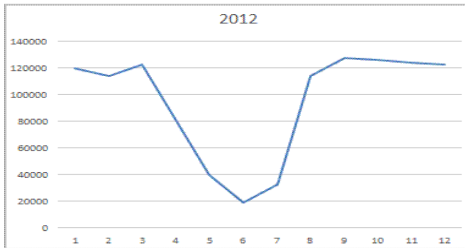
KUVA 45. Sähkönkäytön trendimittaus 2012
