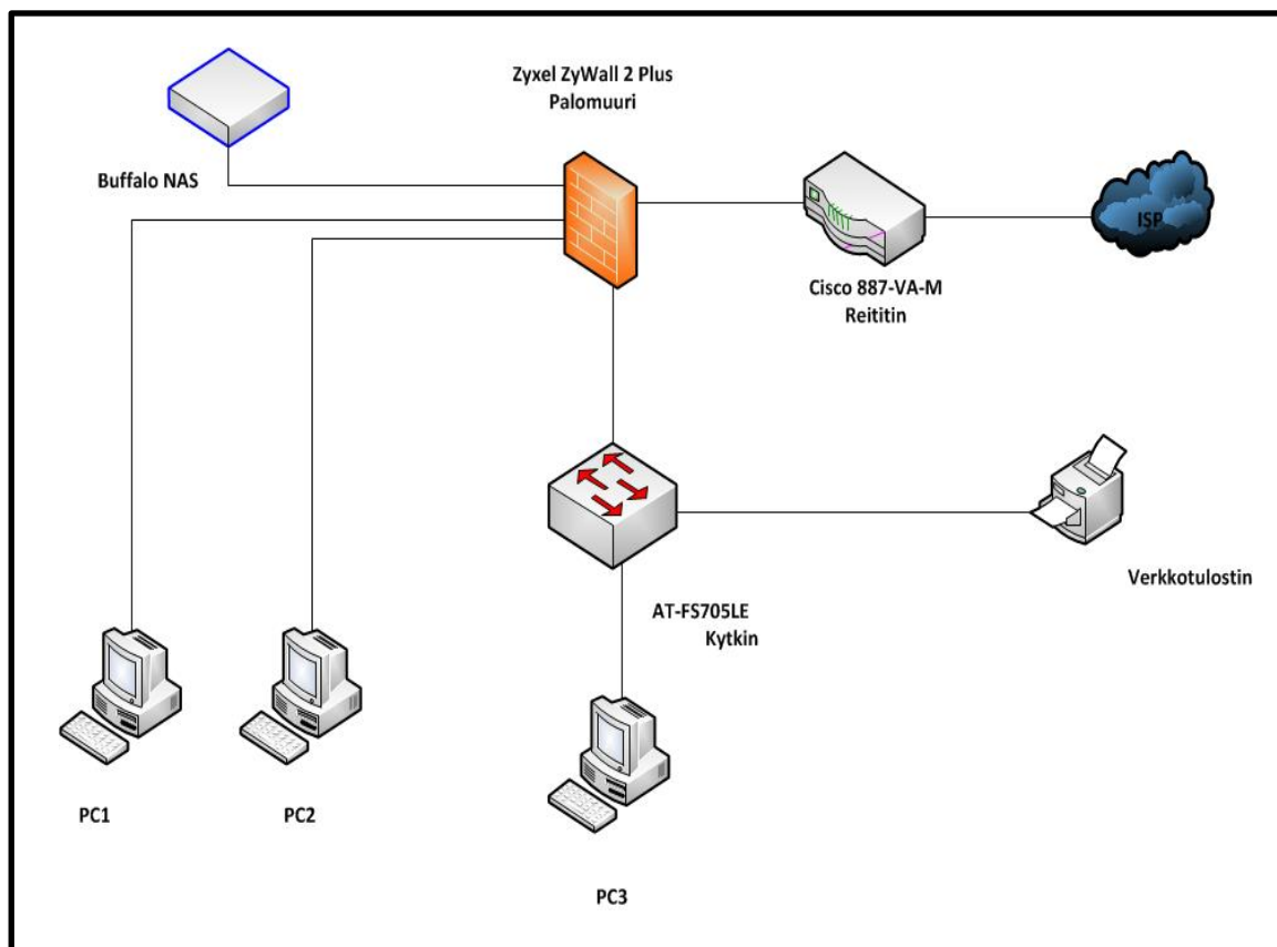
Kuva 6. Hämeen Monitoimitilien verkkokuva
