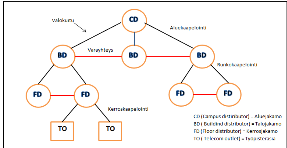
Kuva 1. Yleiskaapeloinnin periaatekuva ( Jaakohuhta 2005, 53)
