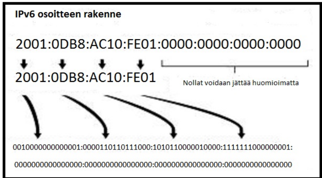
Kuva 4. IPv6-osoitteen rakenne
