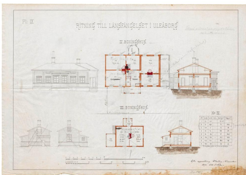
Kuva 19. Rakennuspiirustukset entisen putkan muuttamiseksi henkilökunnan asunnoiksi vuodelta 1893. Rakennuksen vanhassa putkaosassa on kaksinkertainen hirsirunko ja välissä hiekkatäyttö. (Digitaaliarkisto.)
