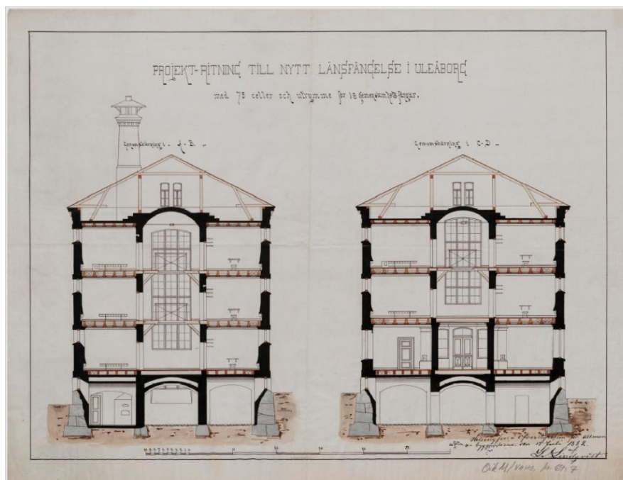
Kuva 12 Vankilan leikkauspiirroksset, laatinut L.I. Lindqvist 1882. Kellarin katossa on kaksoisholvirakenne, jonka sisällä lämmintä ilmaa johdettiin ylempiin kerroksiin metallikanavia pitkin. (Digitaaliarkisto.)
