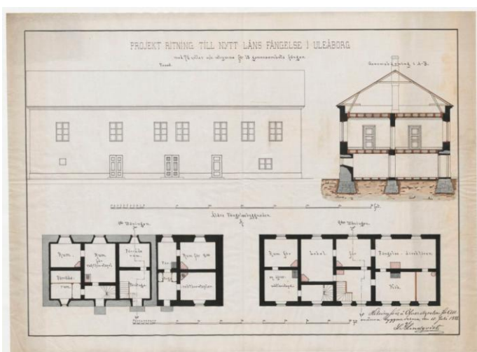
Kuva 17. Rakennuspiirustukset entisen kruununvankilan (Oxens tiernan talo) muuttamiseksi henkilökunnan asunnoiksi. 15.7.1882 L.I. Lindqvist. (Digitaaliarkisto.)
