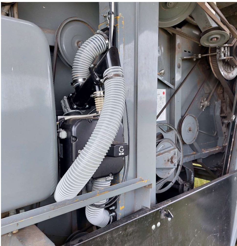
KUVA 8. GrainSensen virtausanalyysointilaite asennettuna
