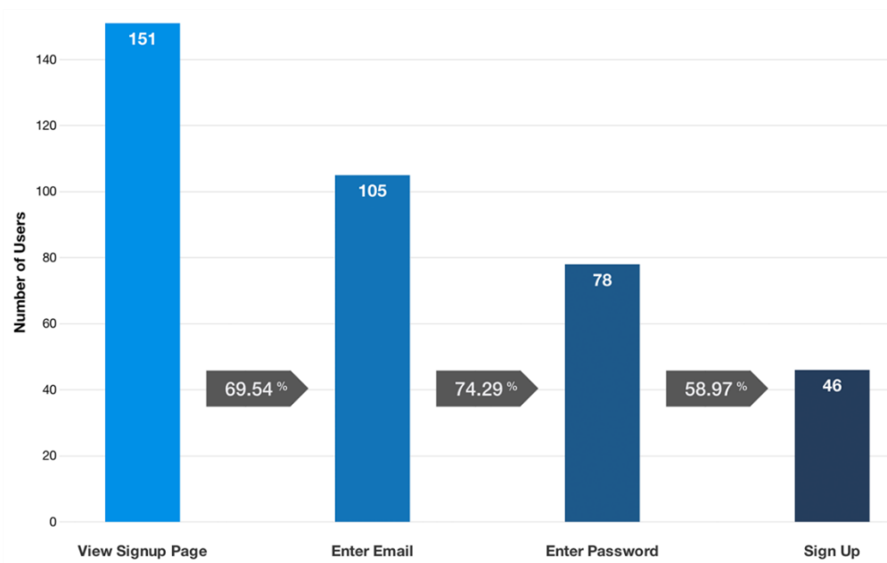
Kuva 10. Esimerkki funnelista.
