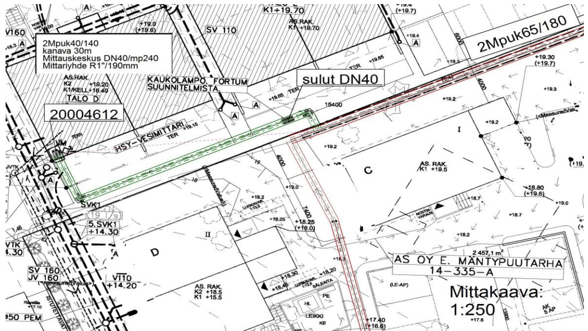
Kuva 4. Trimble NIS-ohjelman suunnittelupuoli. Suunnitelmaan tehty linja korostettu vihreällä välillä. Punaisella värillä oleva linja kuvaa ohjelman aiemmin suunniteltua putkea.
