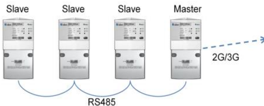
Kuva 12. RS-väylä [13.]
