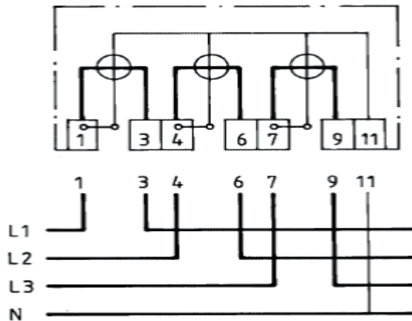
Kuva 1. Suoramittaus [7].
