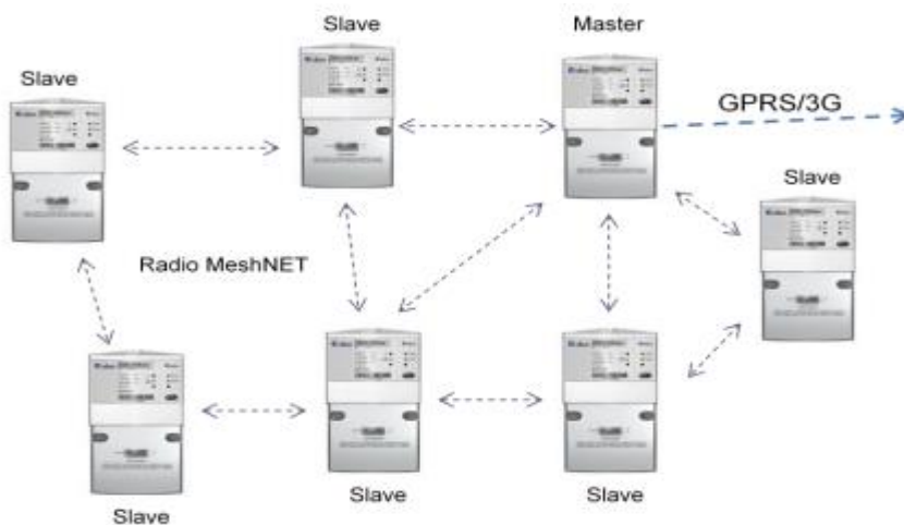
Kuva 11. MESH-radioverkko [13.]
