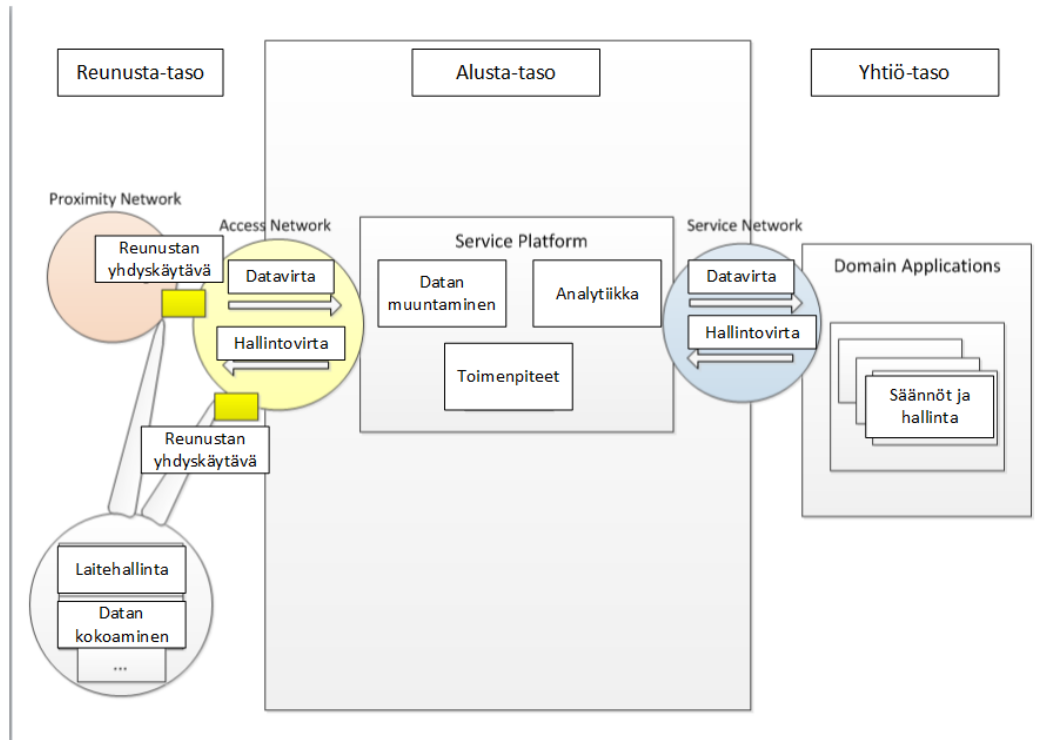
Kuva 5. Kolmitasoinen IIS-arkkitehtuuri (Industrial Internet Reference Architecture 2015, 38)
