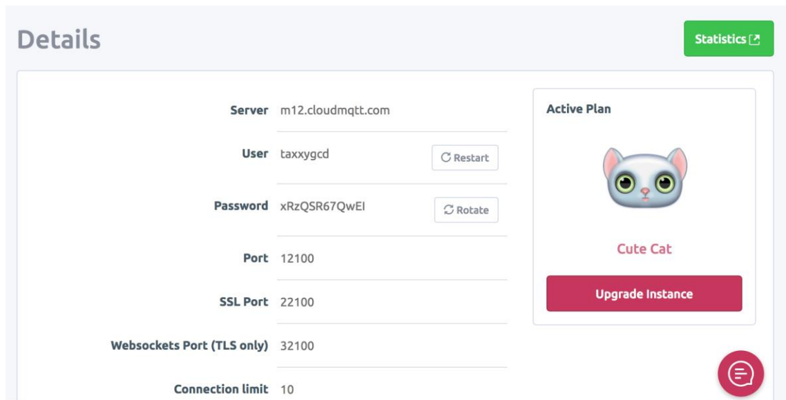
Kuva 12. Instanssien yksityiskohdat. [14].
