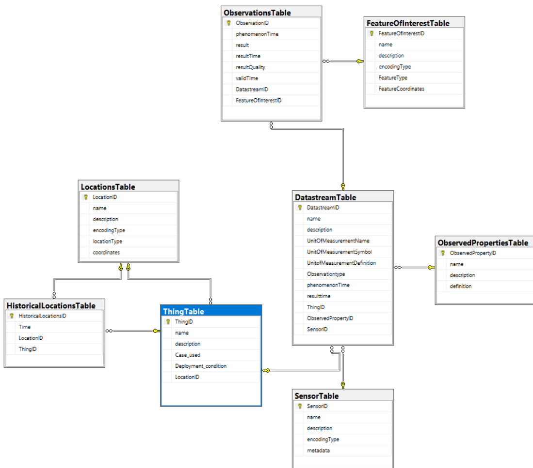
KUVA 10 Lopullinen tietokantarakenne. (Joono Mylly, 2018)
