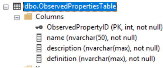
KUVA 6 ObservedPropertiesTable (Joonna Myllys, 2018)
