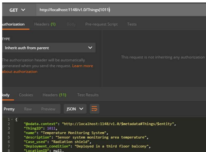
KUVA 12 Yhden objektin haku GET-kutsulla, palautuva data. (Joono Mylly, 2018)
