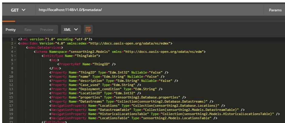
KUVA 13 GET-kutsulla metadatan haku. (Joono Mylly, 2018)
