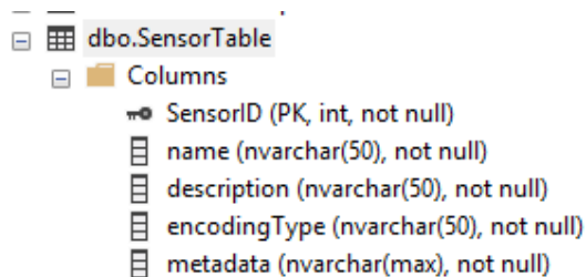
KUVA 7 SensorTable (Joonna Myllys, 2018)
