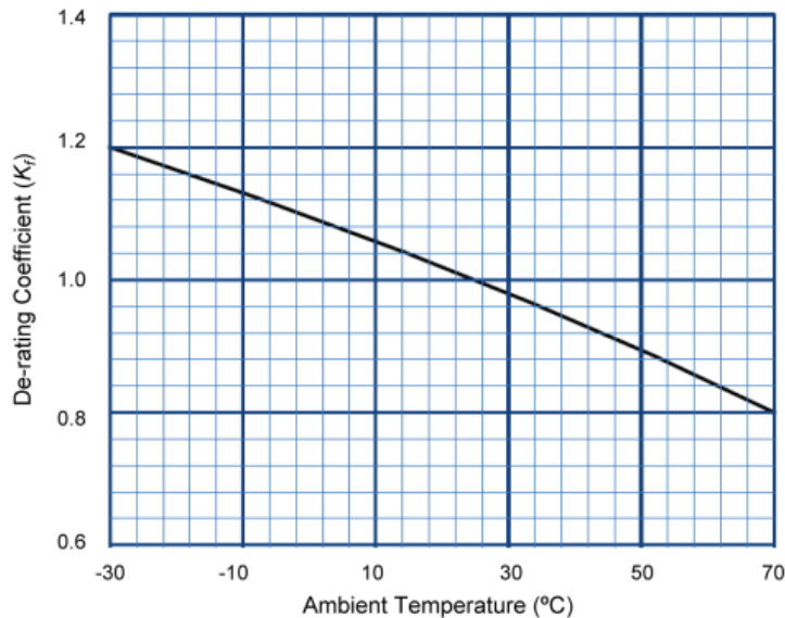
Kuva 9. Lämpötilakerroimen kaavio [23]
