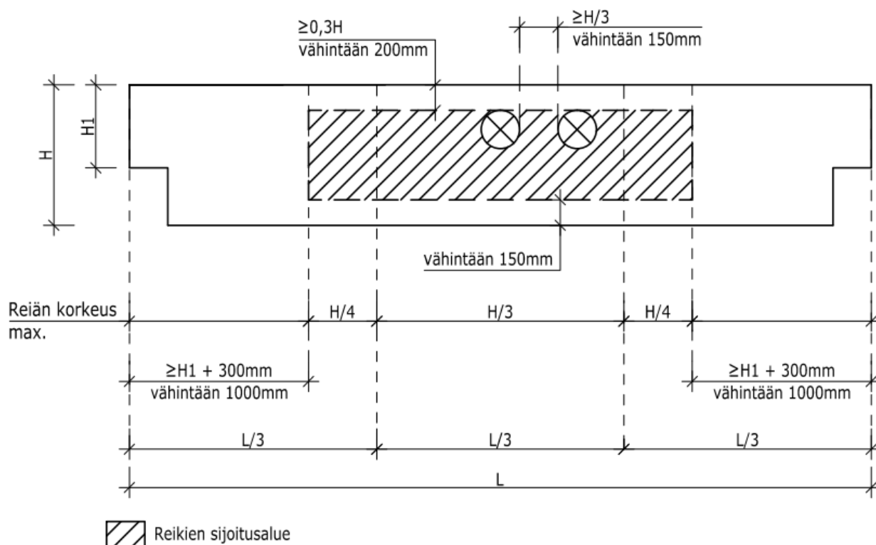
KUVA 2. Päistä lovetun palkin periaatteellinen rei'itysohje (ks. myös lähde 11)
