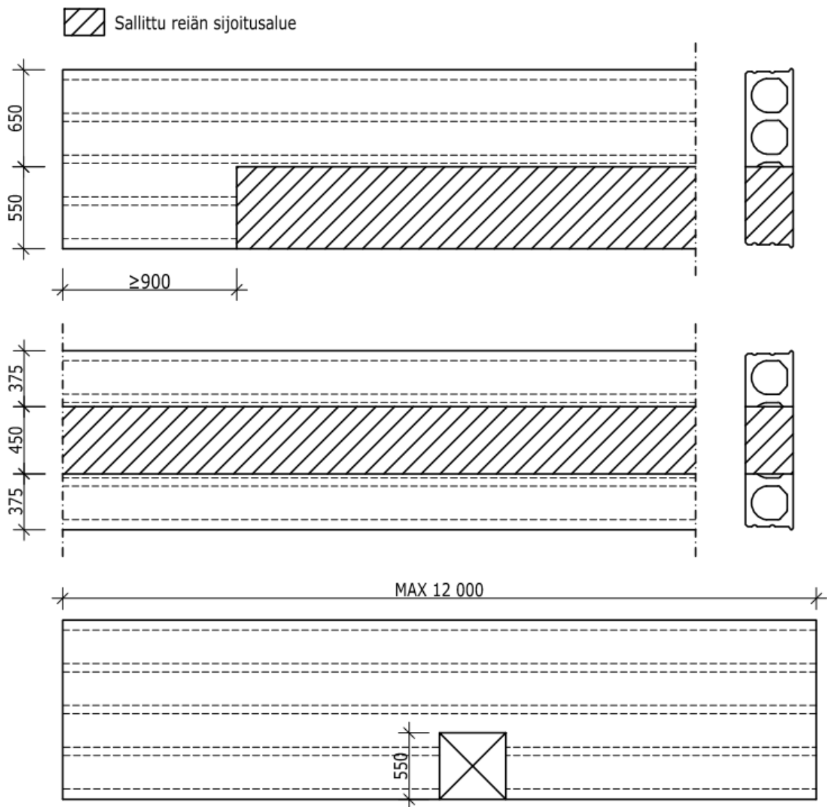
KUVA 4. Nelionteloisen ontelolaattojen periaatteelliset rei'itysohjeet (ks. myös lähde 17, s. 8,10)
