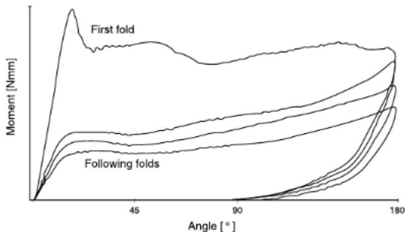
KUVIO 2. Taitettavuusmomentin muutos (Joukio R. & Mansikkamäki S. 1998, 235)
