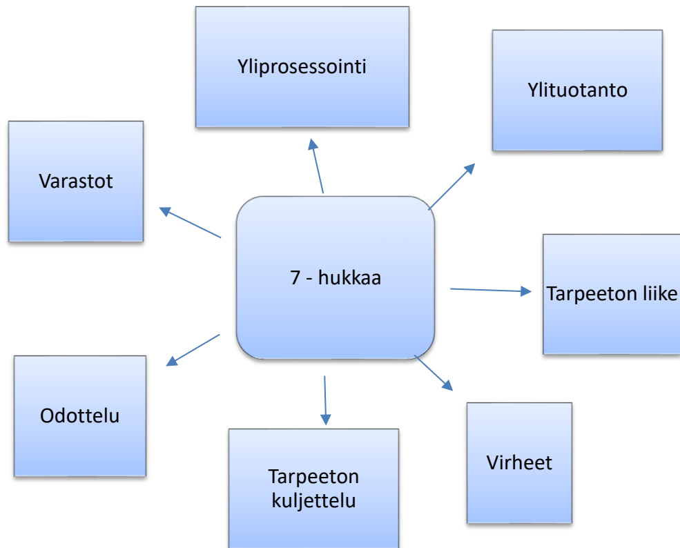
KUVA 4. Lean-mallin 7-hukkaa
