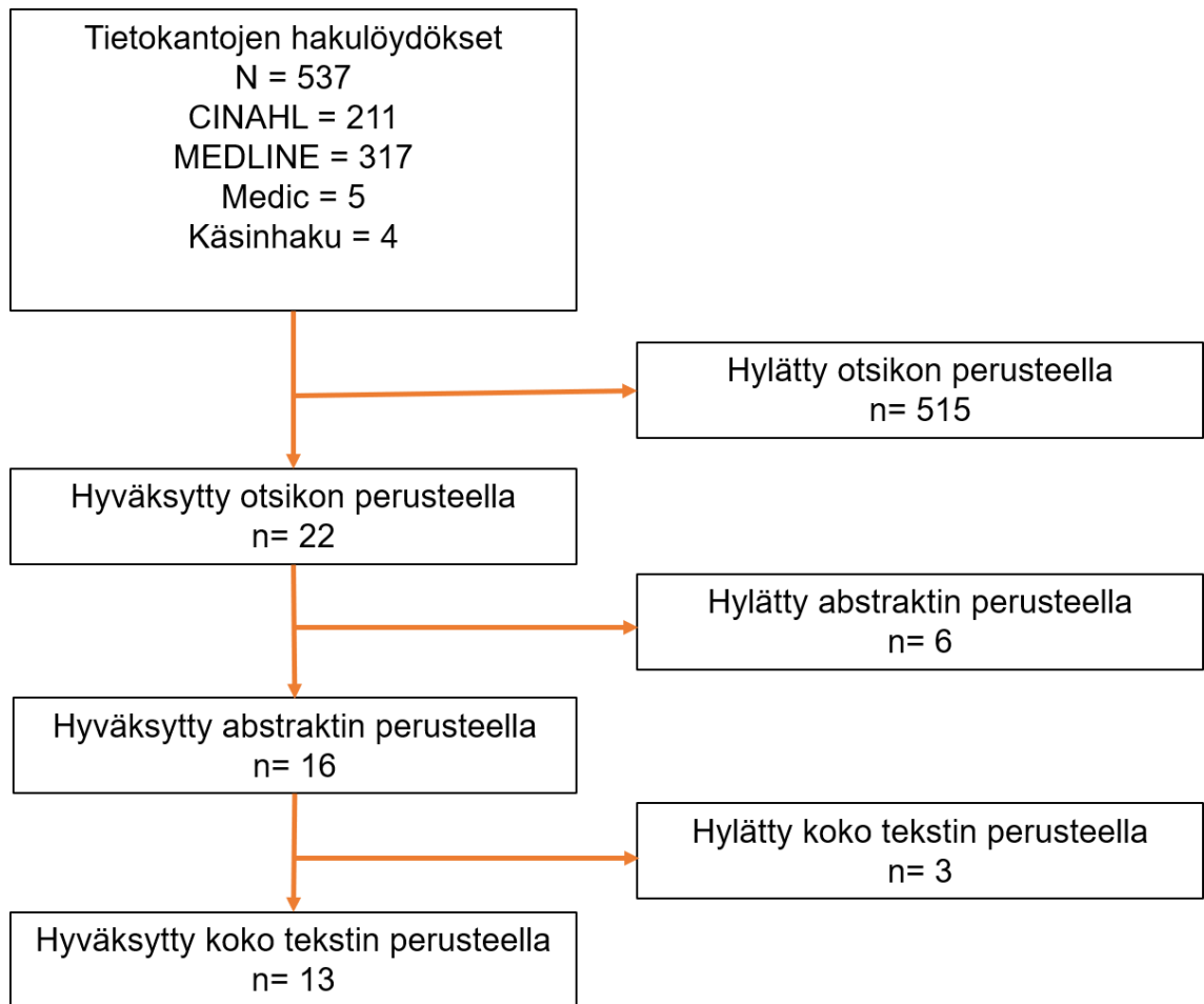
Kuvio 1. Tietokantahaut
