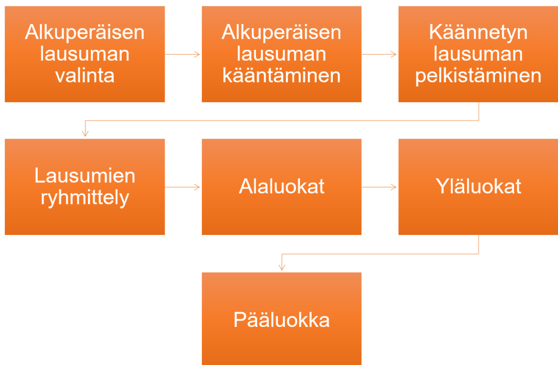
Kuvio 2. Analyysiprosessi
