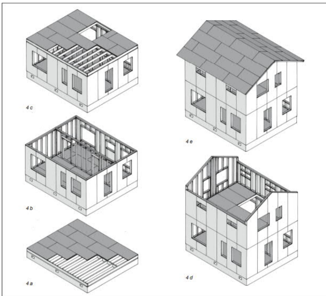
Kuvio 1. Paikalla rakentamisen vaiheet (Viljakainen 2004, 12)
