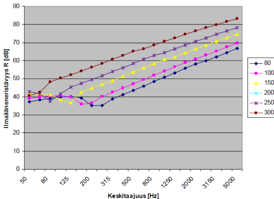
Kuva 9. Ilmääneneristävyys K30 betonilla taajuuden funktiona (Elementtisuunnittelu 2010, 7.)
