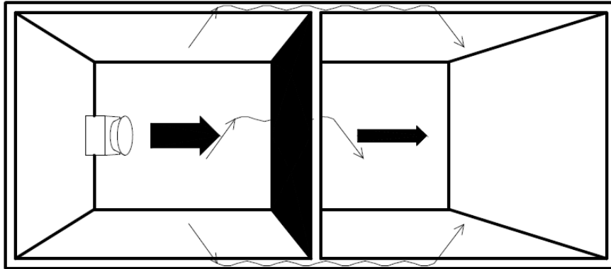
Kuva 7. Ilmaääneneristävyyden mittaus rakennuksessa (Elementtisuunnittelu 2010, 9.)
