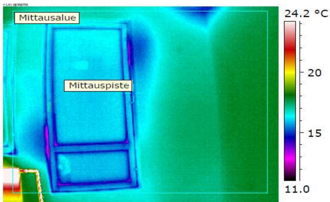
Kuva 10: ranskalaisen parvekkeen oven karmi vuotaa lämpöä./11/
