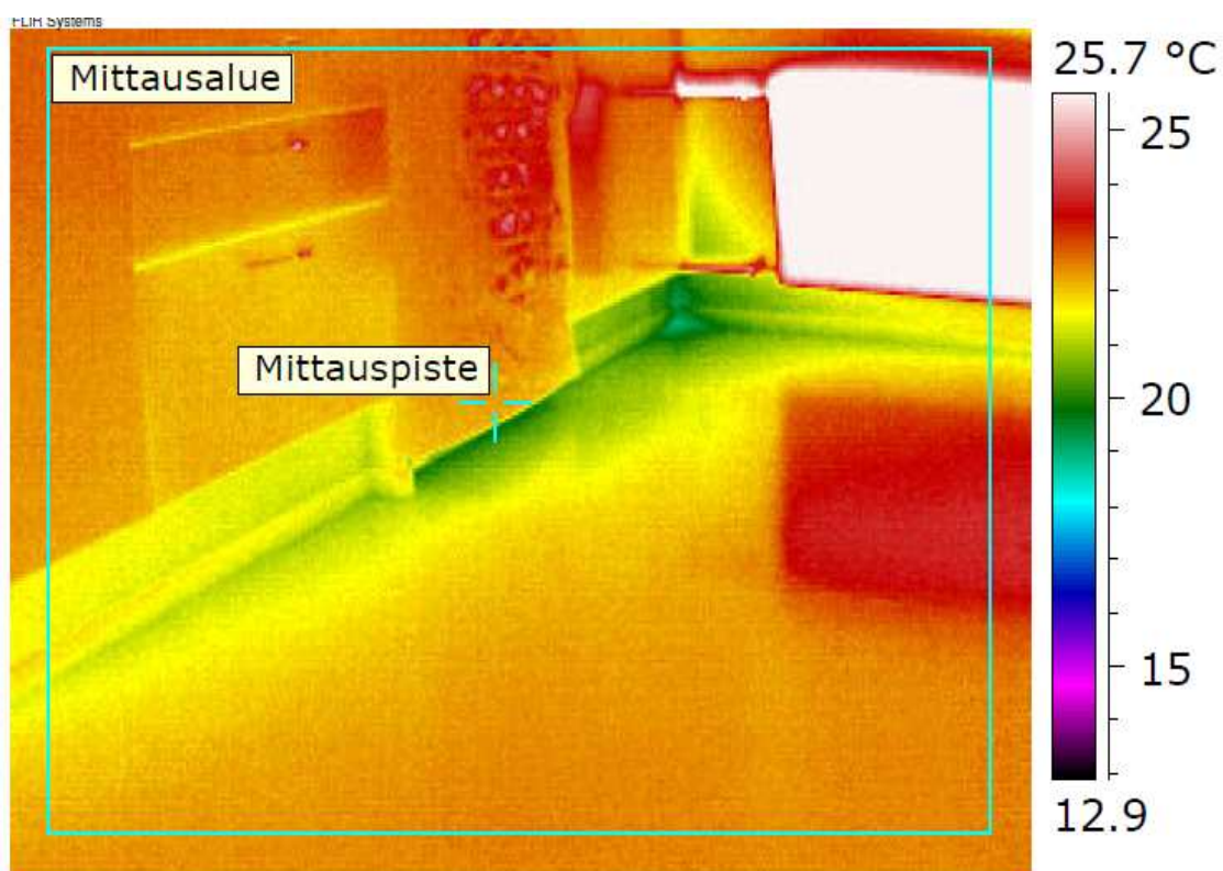
Kuva 11a: Kalusteen ja seinän nurkassa on lämpövuoto./11/
