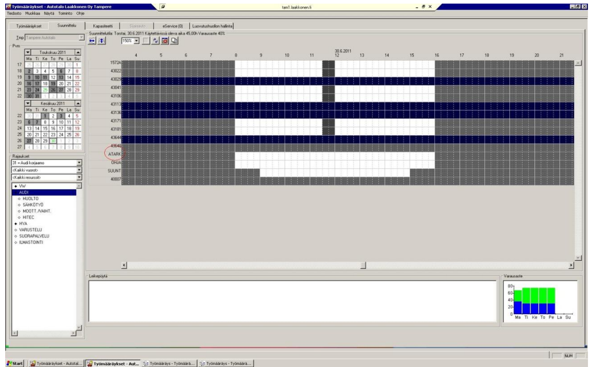
KUVIO 4. Ajanvarauskalenteri
