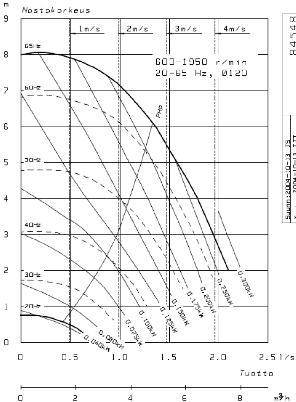
Kuvio 6. Pumpun Kolmeks AE 25/4FC ominaiskäyrät.
