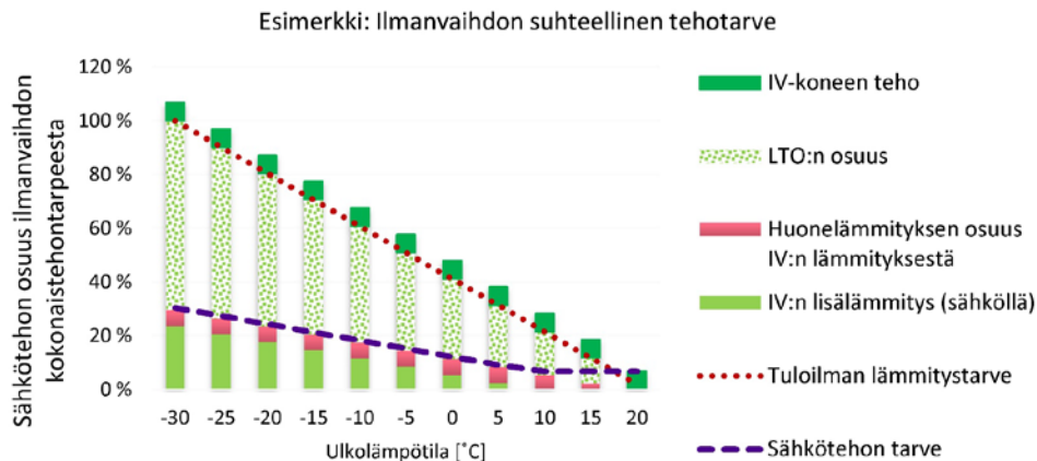
Kuva 5.20 Esimerkki ilmanvaihdon tehotarpeen jakautumisesta. Lämmön talteenoton osuuteen vaikuttaa LTO:n lämpöhyötysuhde ja huonelämmitystarpeen suuruuteen jälkilämmityksen teho. Ilmanvaihdon lämmitystehon tarve vastaa tilannetta, jos kohteessa ei ole koneellista ilmanvaihtoa.
