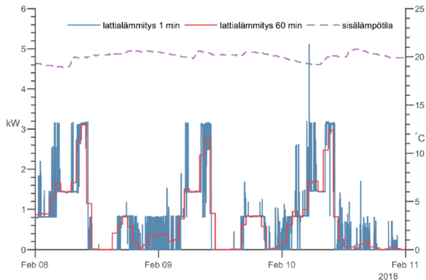
Kuva 5.5 Esimerkki sähkölämmityksiryhmän tehoprofiilista. Ryhmässä kolmen eri tilan lämmitys. Osittain varaava lattialämmitys, asennusteho yhteensä 3,2 kW
