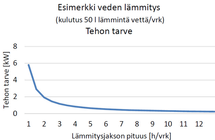
Kuva 5.17 Lämpimän käyttöveden lämmitystehon tarve. Lämmitysjaksoa pidentämällä eli lämpimän käyttöveden varaamisella tehontarve jää pieneksi.
