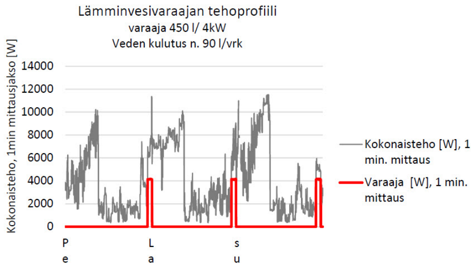
Kuva 5.18 Mittauskohteen lämpimän käyttöveden lämmitysjakso.
