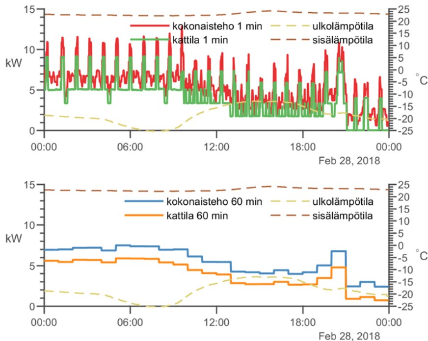
Kuva 5.7 Esimerkki sähkökattilalämmityskohteen tehoprofiilista
