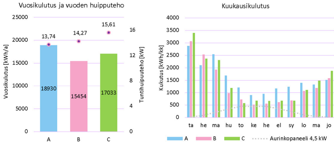
Kuva 2.1. Esimerkki kolmen pientalon energiakulutuksesta vuosi- ja kuukausitasolla. Kohteen A vuosikulutus 18,9 MWh/a ja tunti huipputeho 13,74 kWh/h, kohteen B vuosikulutus 15,4 MWh/a ja tuntihuipputeho 14,27 kWh/h, kohteen C vuosikulutus 17,0 MWh/a ja tuntihuipputeho 15,61 kW.
