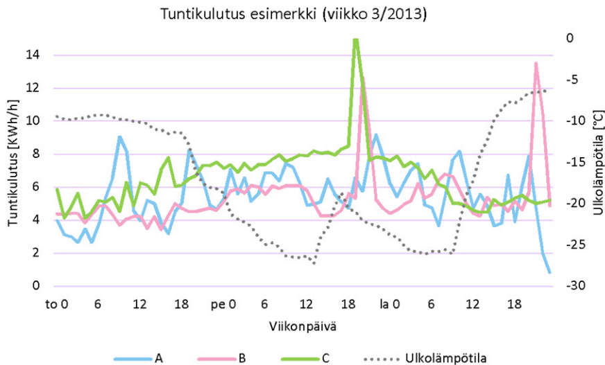
Kuva 2.2 Esimerkki kolmen pientalon energiakulutusesimerkistä verkon huippukulutusaikana. Tuntimittaus.
