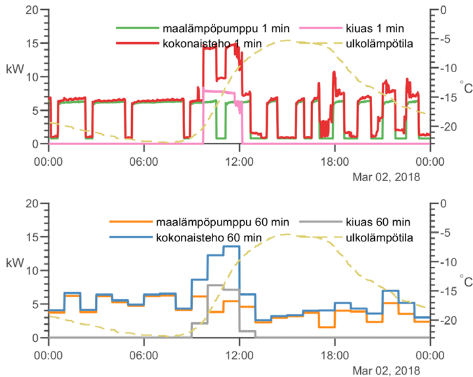
Kuva 5.9 Tehoprofiiliesimerkki. Maalämpö ja sähkökivaas.
