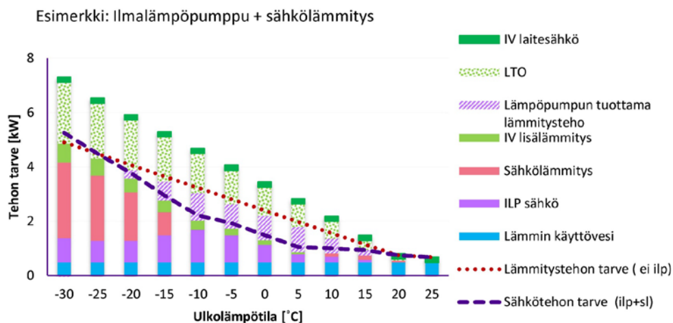
Kuva 5.8 Laskennallinen sähkötalon tarve sähkölämmitys + ilmalämpöpumppuratkaisussa. (Esimerkkikohte A_{\text{netto}} = 125 \text{ m}^2 )
