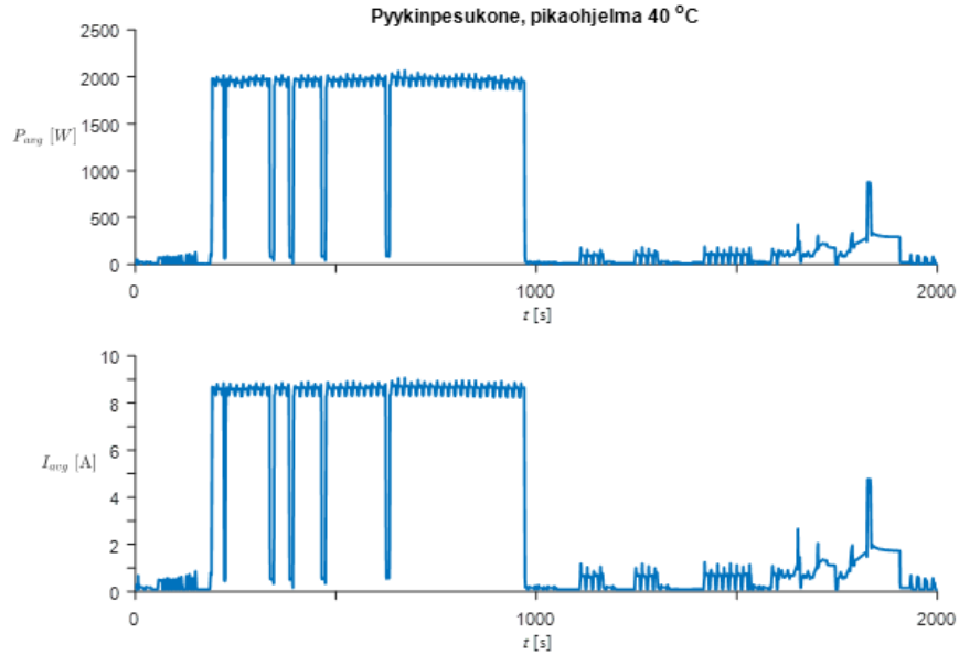
Kuva L1.2 Esimerkki pesukoneen tehoprofiilista.
