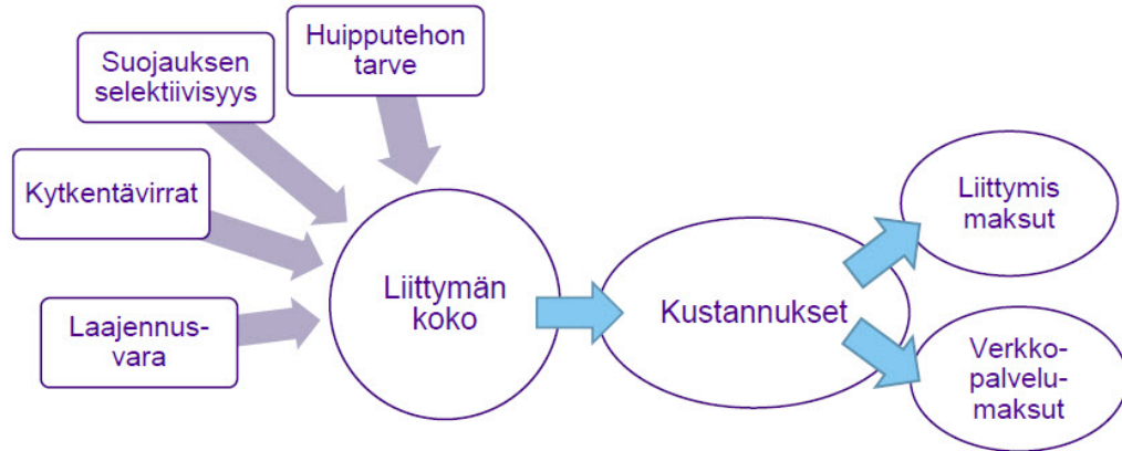
Kuva 3.4 Liittymän pääsulakkeiden suuruuteen vaikuttavia tekijöitä.
