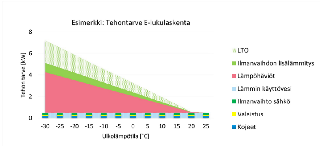
Kuva 3.2 Pientalon ( A_{\text{netto}} = 125 \text{ m}^2 ) tehontarvejakauma energiatehokkuuslaskennan arvoilla. LTO kuvastaa ilmanvaihdon lämmöntaloteenoton vaikutusta tehontarpeeseen.
