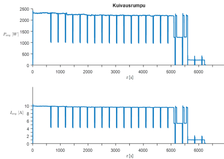
Kuva L1.3 Esimerkki kuivausrummun tehoprofiilista.
