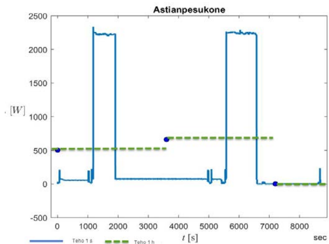
Kuva 5.21 Astiapesukoneen tehoprofiili pesuohjelman aikana.
