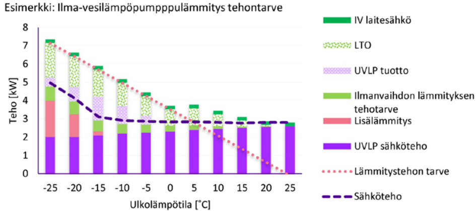
Kuva 5.12 Esimerkki laskennallisesta sähkötehon tarpeesta. Esimerkissä käyttöveden lämmitys on oletettu jatkuvaksi. (Esimerkkikohde A_{\text{netto}} = 125 \text{ m}^2 )
