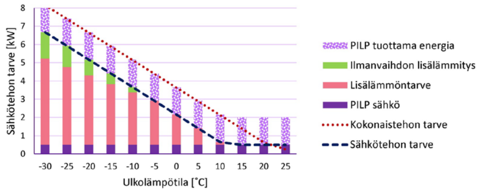
Kuva 5.13 Laskennallinen sähkötehon tarve PILP-ratkaisussa. (Esimerkkikohte A netto = 125 m 2 )
