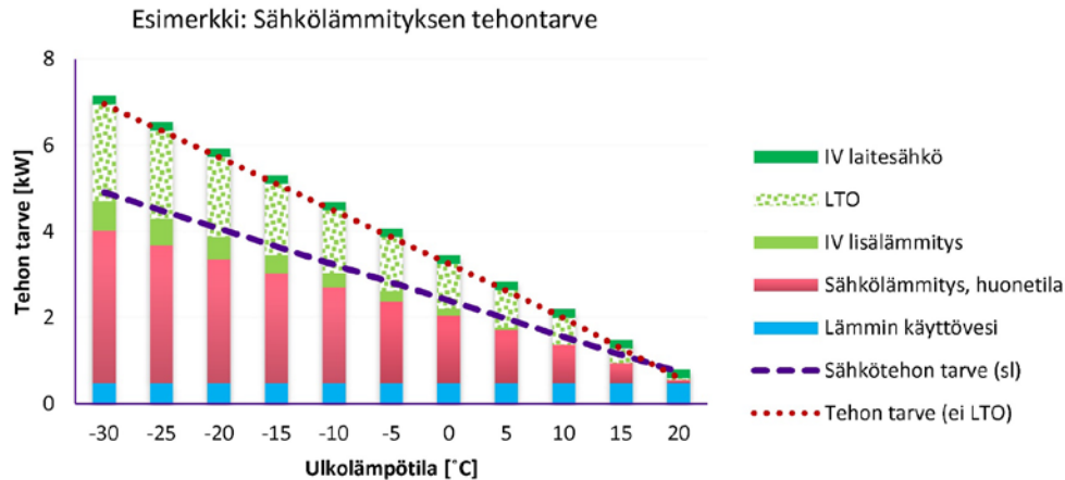
Kuva 5.4 Sähkölämmitysratkaisun tehontarve. (Esimerkkikohde A_{\text{netto}} 125 \text{ m}^2 ). LTO-osa kuvastaa ilmanvaihdon lämmön talteenoton vaikutusta tehotarvetta pienentävästi.
