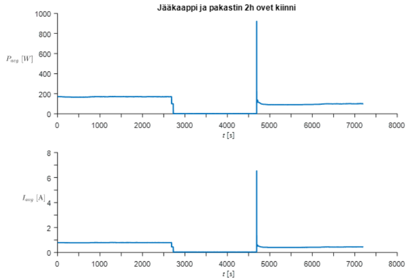
Kuva L1.4. Jääkaapin tehoprofiili
