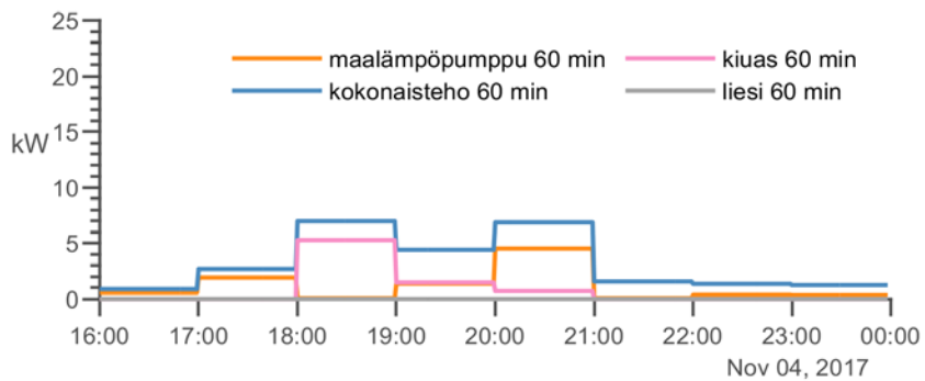
Kuva 5.11 Pilottikohteessa mitattu sähkötehon profiili. Ylemmässä kuvassa laitekohtaiset profiilit koko vuorokauden ajalta ja alemmassa klo 16:00 alkaen.
