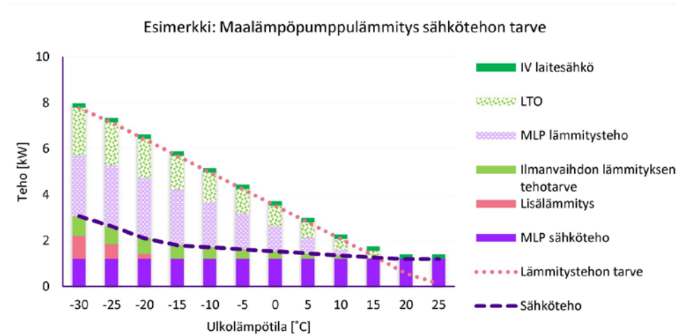
Kuva 5.10 Esimerkki maalämpöratkaisun sähkötehon tarpeesta (Esimerkkikohde A_{\text{netto}} 125 m 2 )
