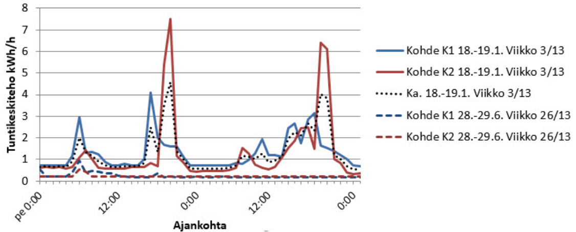
Kuva 5.16 Kahden kaukolämpökohteen sähkönkulutusesimerkki talvi- ja kesäaikaan. Ka= kulutuksen keskiarvo.
