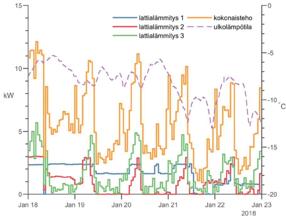
Kuva 5.6 Esimerkki aikaohjatusta lattialämmityksestä. Varausaika on ohjattu ensisijaisesti aamuyön aikaan ja veden lämmitys iltayöhön.
