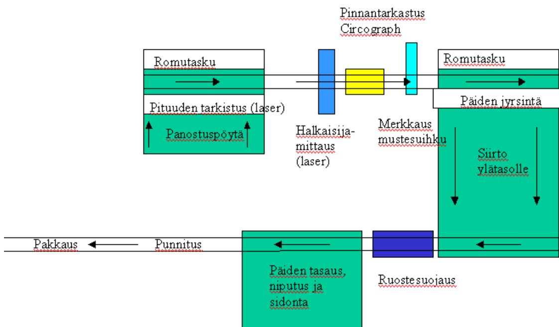
Kuva 2. BBF – tarkastuslinjan layout (Ovako, sisäinen tietojärjestelmä)
