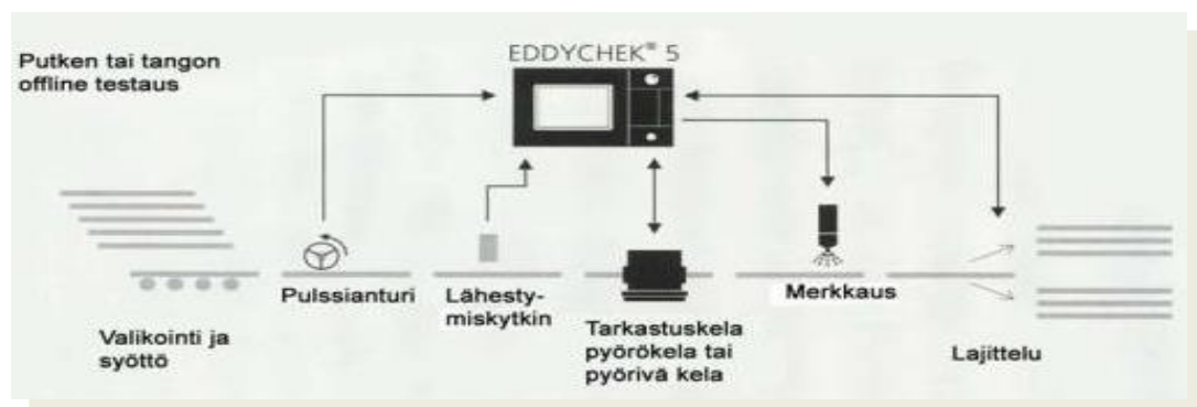
Kuva 15. Pinnantarkastuslaitteiston säätöperiaate
