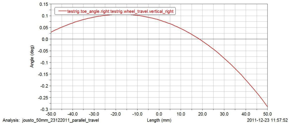
Kuvio 11. Oikean eturenkaan aurauksen muutos joustomatkan suhteen.
