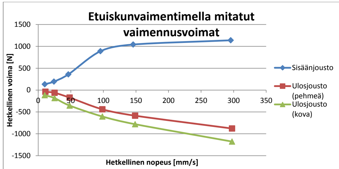
Kuvio 7. Etuskunvaimentimella testipenkissä mitatut vaimennusvoimat ulos- ja sisäänjoustossa.
