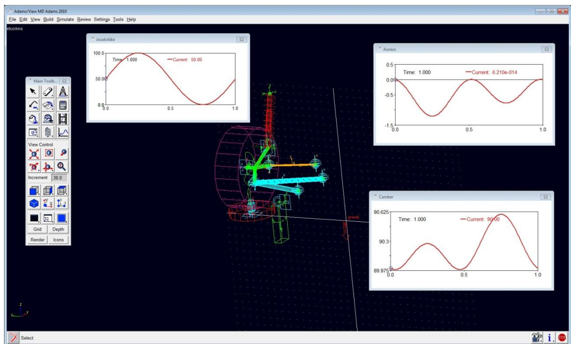
Kuvio 9. Etutuenta mallinnettuna Adams/AView-ohjelmalla.
