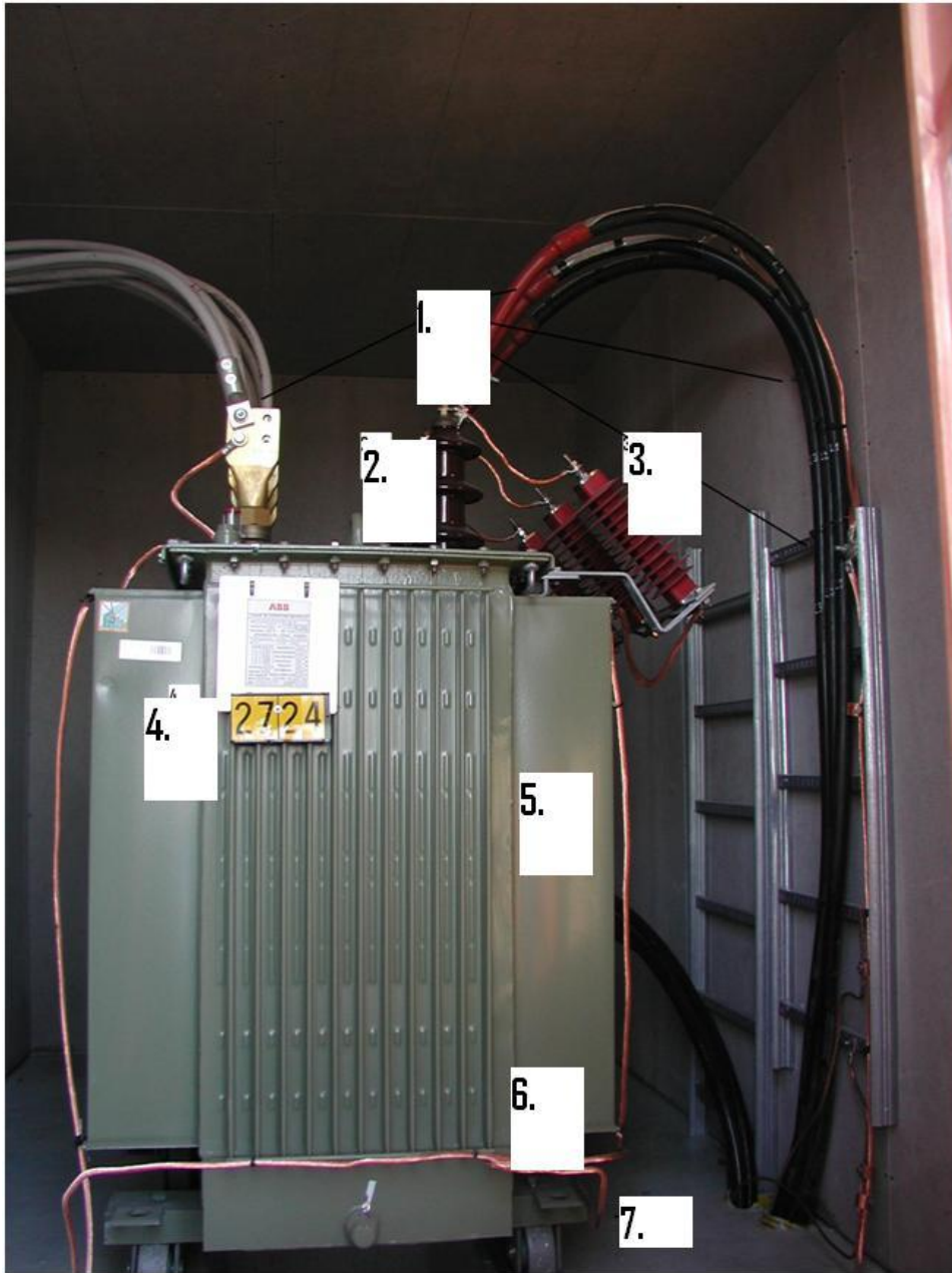
Kuva 4. Muuntaja kiinteistössä /13/
