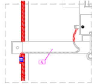
DET. 4 MUUNTAJAN MAADOITUS, MAADOITUSKOHTIÖ SÄILIÖN ALAOSASSA
