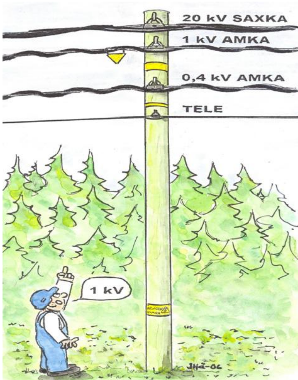
Kuva 11. Yhteiskäyttöpylväänmerkinnät /30/
