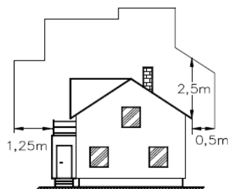
Kuva 8. Pj-johdosten etäisyydet rakennuksista /2/
