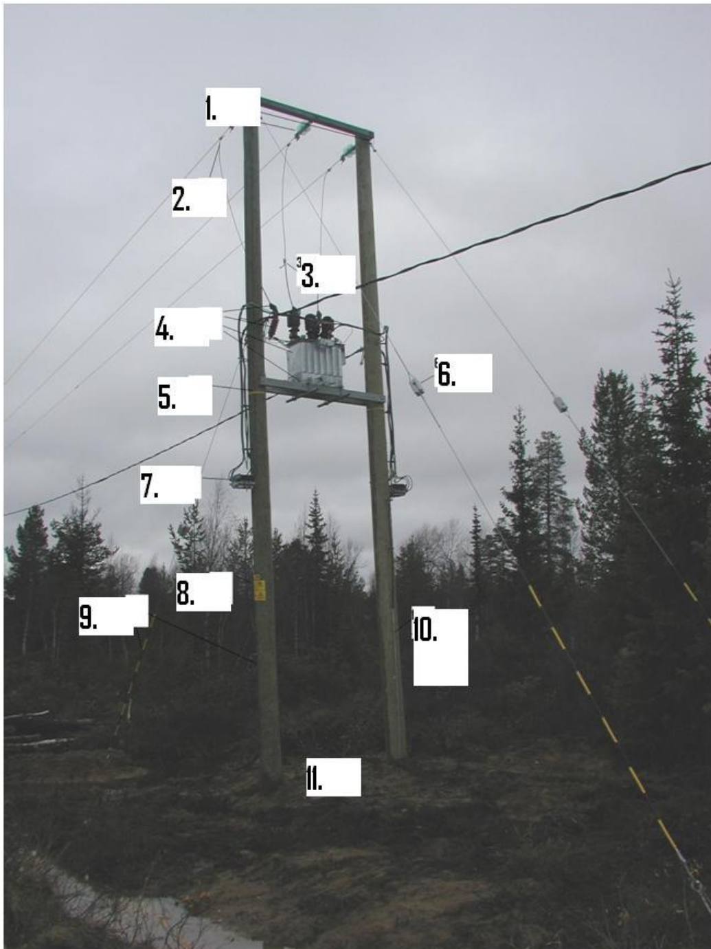
Kuva 2. Tarkastuskohteita pylväsmuuntamolla /13/
