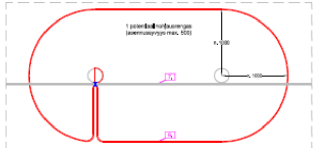
DET. 6 LEIKKAUS A-A 1 POTENTIAALINOHJAUSRENGAS
