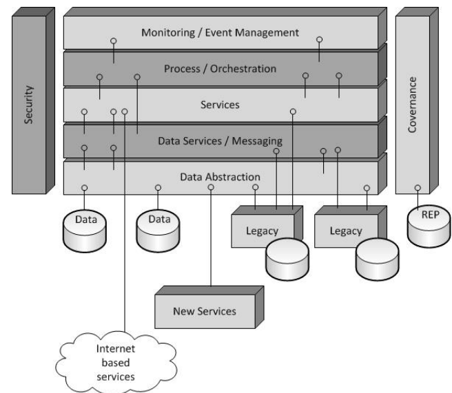
Fig. 4 SOA Metamodel
