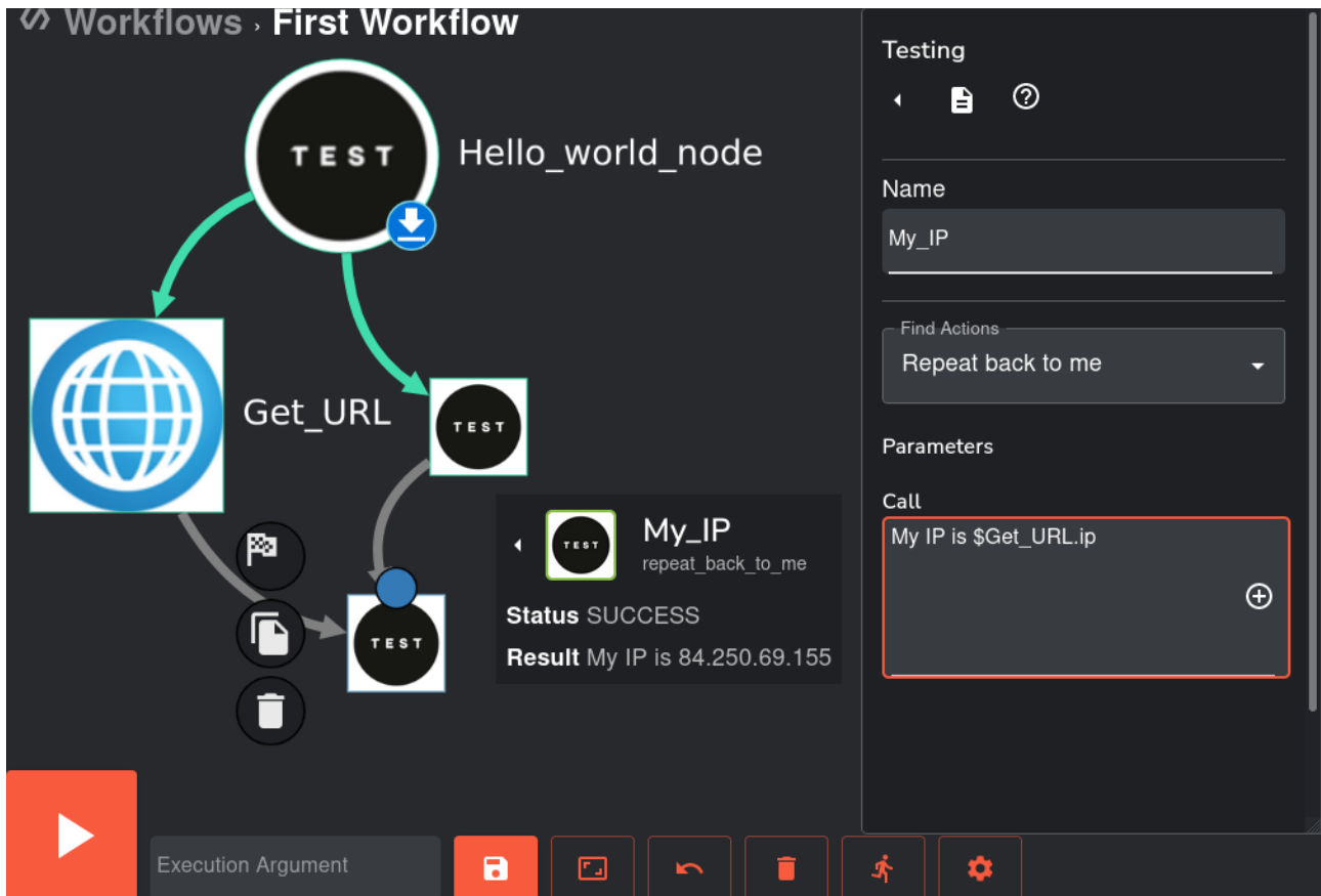
Kuvio 12. Shuffle My_IP ja onnistunut suoritus
