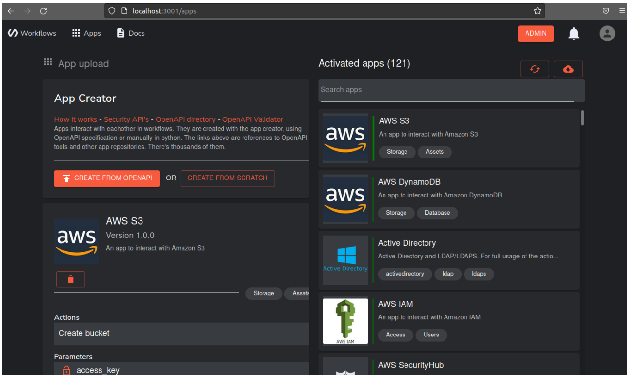
Kuvio 6. Shuffle Apps-näkymä, lista applikaatioista
