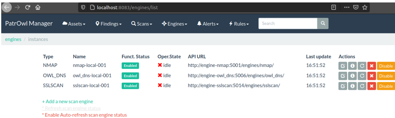
Kuvio 22. PatrOwl ennakkoon konfiguroidut moottorit
