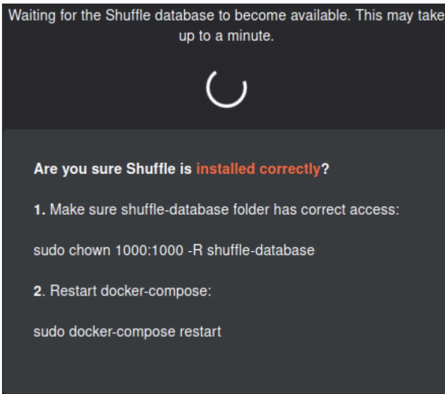
Kuvio 3. Shufflen asennuksen aikana ilmennyt ongelma
