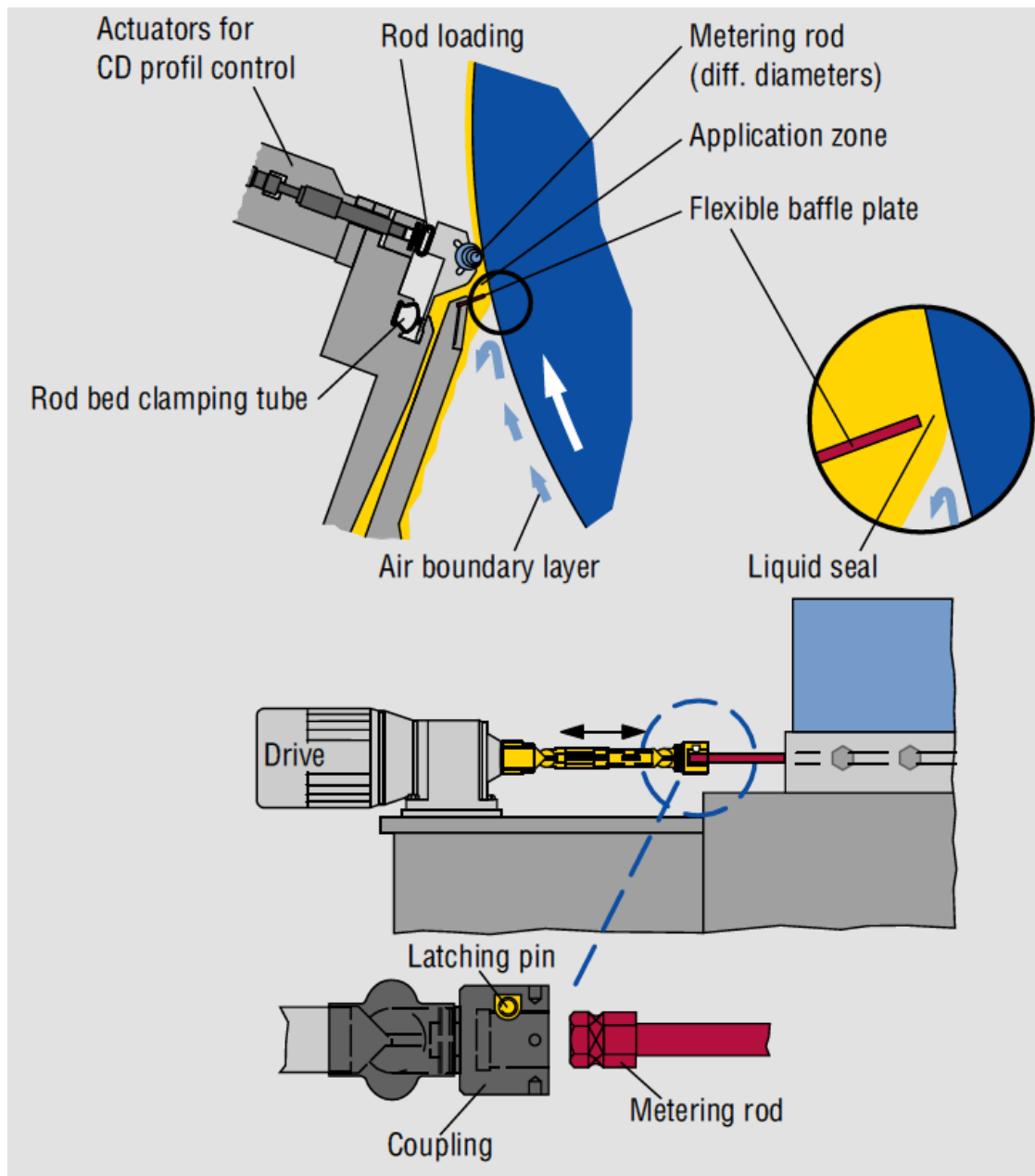
Kuva 2.1 Voith Paper: in Speed Sizer filmipäälystyn sauvakaavinnalla ja esimerkki sauvan kytkennästä moottoriin (Voith Paper, s. 3, 5)
