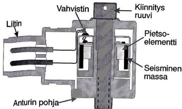
KUVA 3. Kiihtyvyyksanturin rakenne (6, s. 46)
