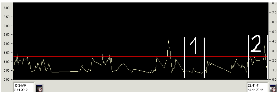
KUVA 11. Paperinjohtotela 60 HP:n nopeuden RMS 3–600 Hz, 11 päivän trendi
