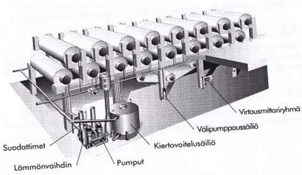
KUVA 1. Kiertovoitelujärjestelmän rakenne (7, s. 227)
