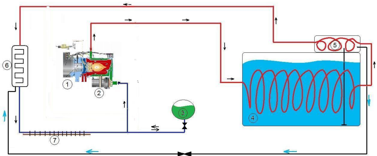
KUVA 3. Lämmitysjärjestelmä (ks. 5)
