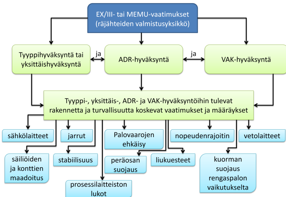
KUVA 2. Ajoneuvon hyväksyntävaiheet
