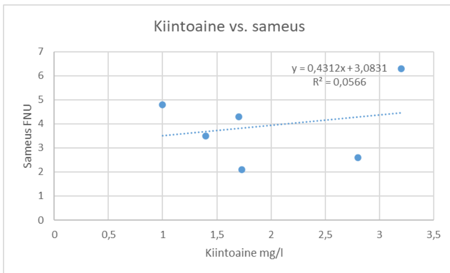
KUVA 10. Kiintoainepitoisuuden ja sameuden välinen korrelaatio syksyllä 2020
