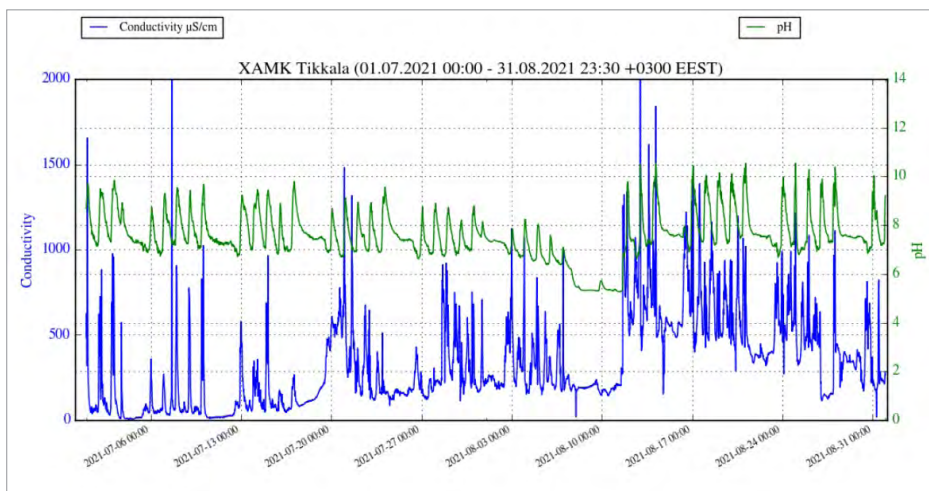
KUVA 6. Heinä–elokuun mittaustulokset EHP Environment Oy:n anturien osalta.
