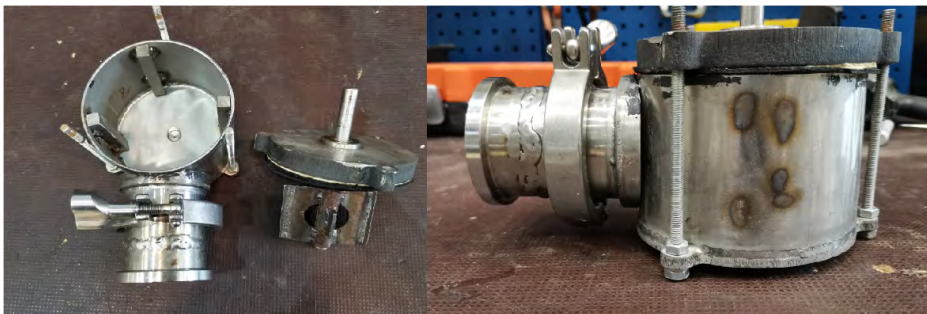
KUVA 2. Pieni sekoitin kaasudispersiokokeisiin. Sekoitinta voidaan ajaa akkukäyttöisellä porakoneella, ja se on mahdollista ottaa mukaan tehtaalle. (kuva Antti Pappinen)
