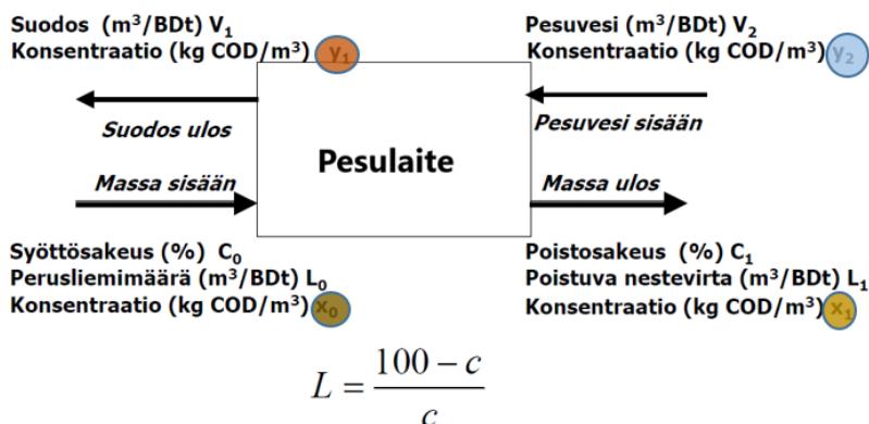
KUVA 5 Yksittäisen pesurin tasemalli, jossa mitattavat pitoisuudet ympäröity (kuva Riku Kopra).
