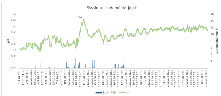
KUVA 3. Sade ja pH-arvon muutos syyskuussa 2020
