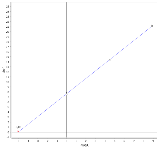
KUVA 3. Kalibrointisuora lyijyn mittaukselle vesinäytteestä (kuva Marjatta Lehesvaara)
