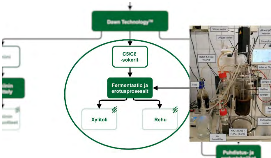
KUVA 2. Fermentaatiokokeen prosessilaitteisto (Kuva Vogelbusch)
