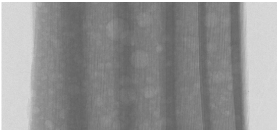
KUVA 1. Yksityiskohta tomografiakuvasta, jossa läpivalaistunutta mäntyä ja epoksiliimaa (kuva Olli Paajanen)
