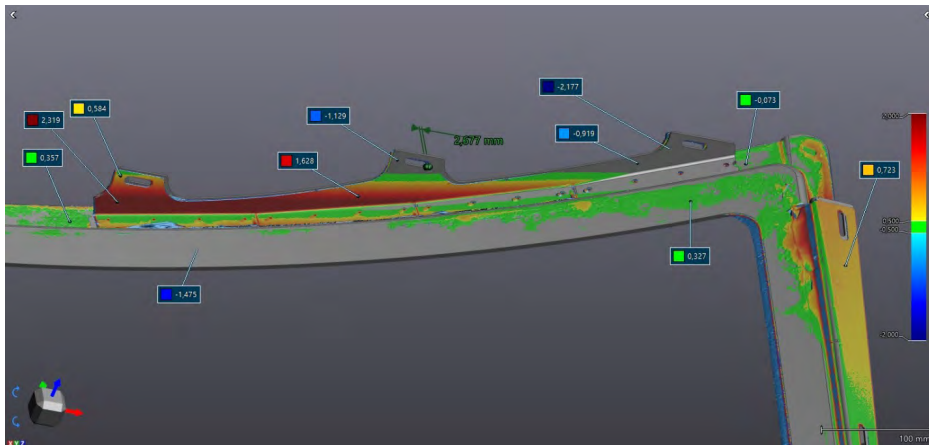
KUVA 6. Mittatarkkuuden tarkastelu väärävärिकartan avulla. Skannattu data ja CAD-referenssi on sovitettu päällekkäin. Positiivinen lukema tarkoittaa, että skannattu data on CAD-mallin edessä ja negatiivisella päinvastoin (kuva Mikko Nykänen).
