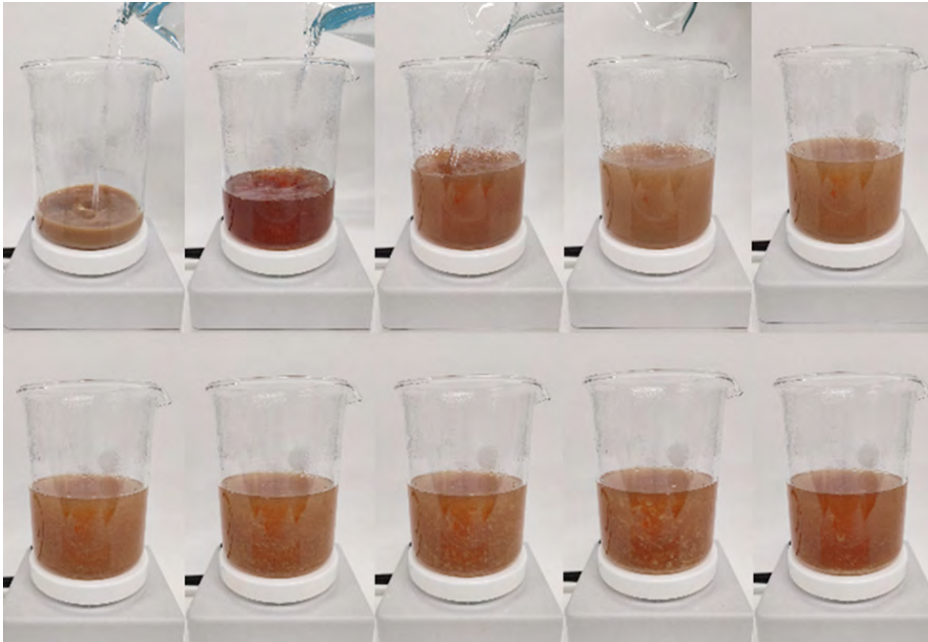
KUVA 1. Alipainehaihdutetun esihydrolysaatin etanolisaostuksen eteneminen (kuva Lotta Pirinen).
