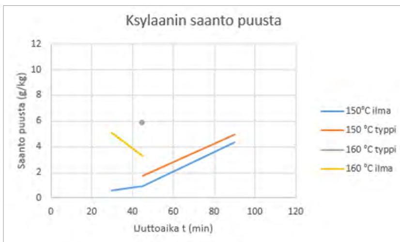
KUVA 6. Ultrasuodatettujen ja etanolisoitettujen näytteiden ksylaanisaannot kilosta kuivaa puuta
