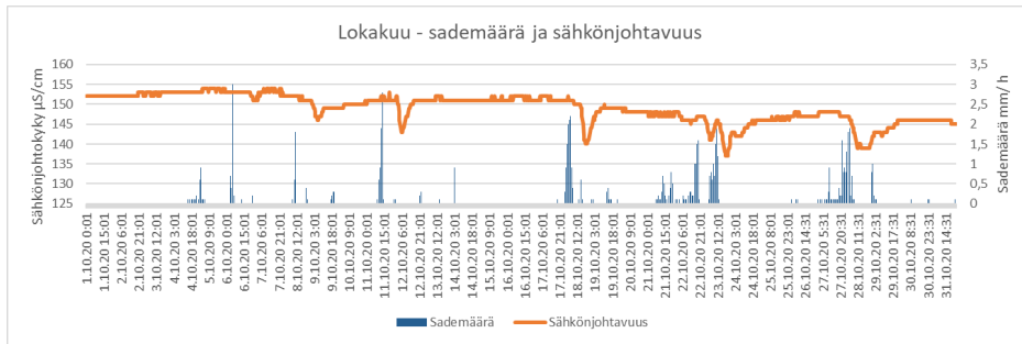
KUVA 2. Lokakuun 2020 sateet ja sähkönjohtavuuden muutos
