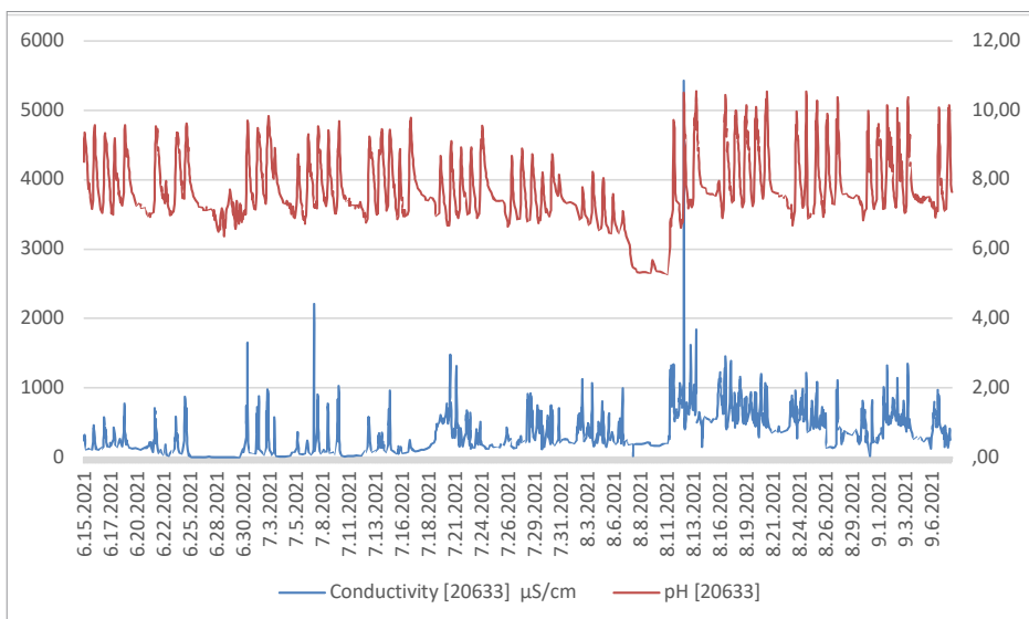
KUVA 7. EHP Environment Oy:n asentamien Ponsel-anturien mittaustulokset 15.6.–8.9.2021.
