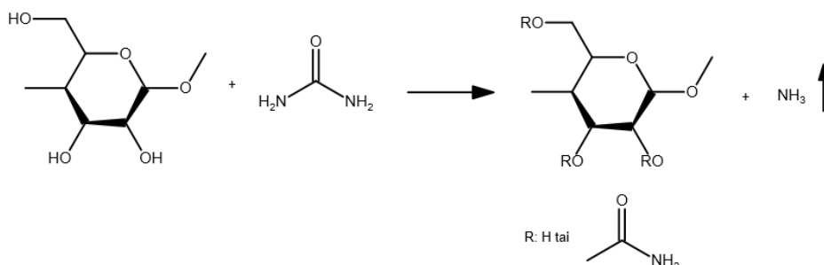
KUVA 1. Selluloosan ja urean reaktio karbamaatioreaktiossa (Kuva Noora Haatanen)
