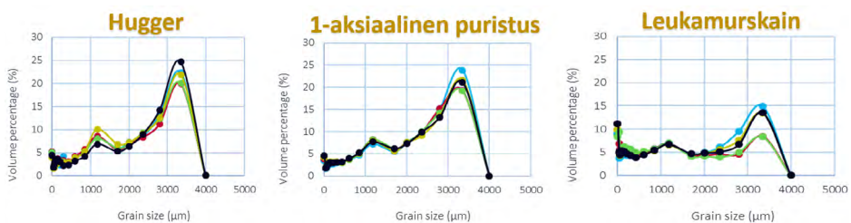
KUVA 5. Partikkelikokojakaumat Hugger-murskaimella, leukamurskaimella ja yksiakiaalisten puristuskokeiden avulla hienonnetuista kivit tuotteista (kuva Niina Paasovaara).
