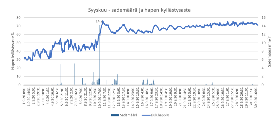
KUVA 6. Sademäärä ja hapen kyllästysaste syyskuussa 2020
