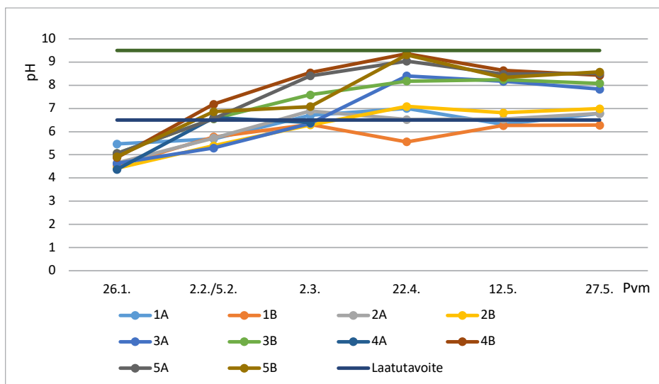
KUVA 3. Tiekolonnikokeen suotovesien pH:n mittaustulokset ja laatutavoite.
