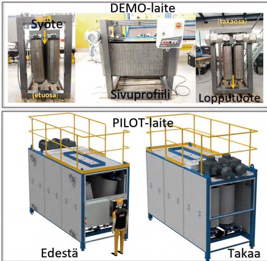
KUVA 1. Yläosassa kuvasarja (kuvat Niina Paasovaara) Hugger-laitteen demoversiosta ja alaosassa suunnitteluvaiheen kuvat pilot-mittakaavan Hugger-laitteesta.
