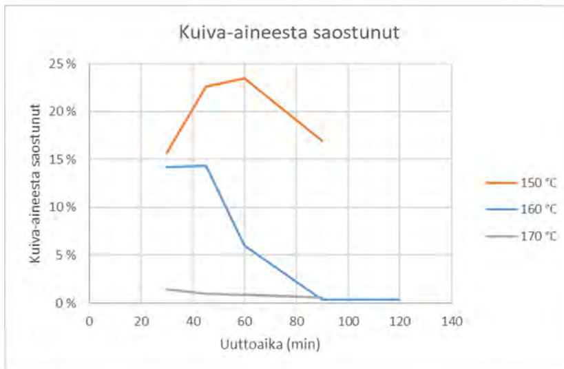
KUVA 3. Alipainehaihdutettujen ja etanolisaostettujen hydrolysaattinäytteiden kuiva-ainesannot alkuperäisen hydrolysaatin kuiva-aineesta.
