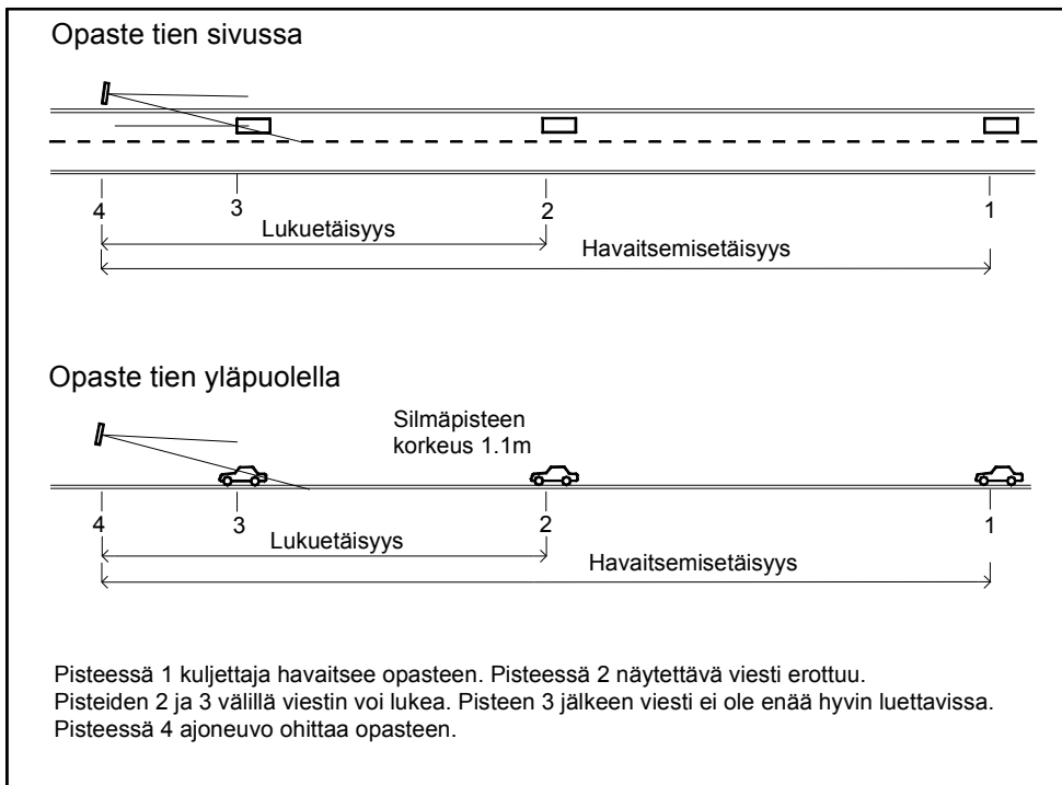
Kuva 1. Itsevalaisevan vaihtuvan opasteen luku- ja havaitsemisetäisyys.
