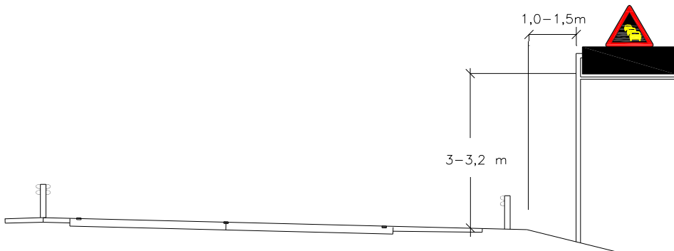
Kuva 14. Esimerkki varoitusmerkin ja tekstillisen kilven yhdistelmän sijoittamisesta nelikaistaisella keskikaidetiellä (pientareen leveys yli 1,5 m). Yhdistelmä sijoitetaan ajoradan yläpuolelle vilkasliikenteisillä teillä.
