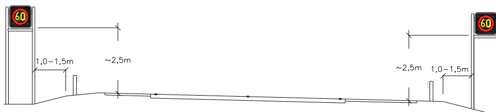
Kuva 3. Esimerkki vaihtuvien nopeusrajoitusmerkkien sijoittamisesta nelikaistaisella keskikaistalla varustetulla tiellä (pientareen leveys yli 1,5 m).
