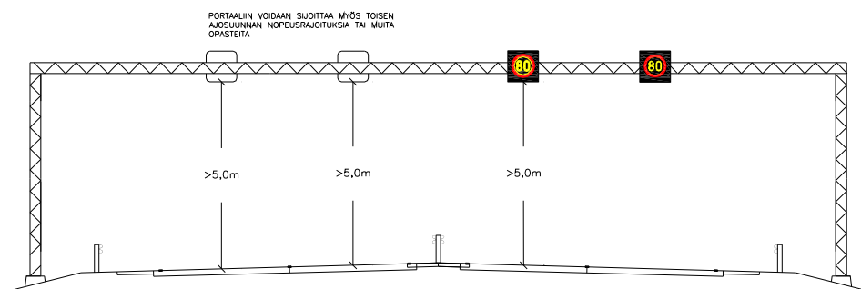
Kuva 4. Esimerkki vaihtuvien nopeusrajoitusmerkkien sijoittamisesta nelikais- taisella keskikaidetiellä.
