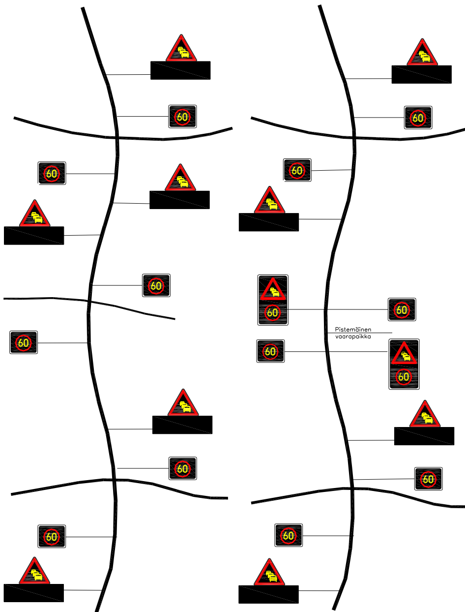
Vaihtuvien opasteiden periaateratkaisu tiejaksolla, jolla esiintyy reittiohjauksen tarvetta
