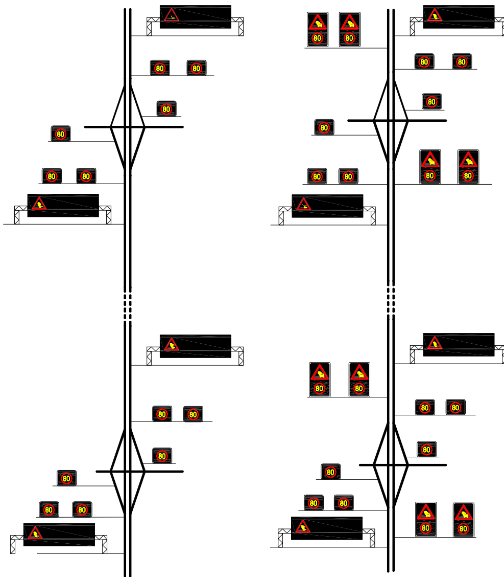
Kuva 21. Vaihtuvat opasteet nelikaistaisella keskikaistalla varustetulla tiejaksolla: vasemmalla vaihtuvien opasteiden perusratkaisu ja oikealla vaihtuvien opasteiden periaateratkaisu tiejaksolla, jolla esiintyy suuresta liikennemäärä aiheutuvia ongelmia. (Merkkien sijoitusperiaatteita on kuvattu luvuissa 2.7, 5.2.2, 11.1 ja 11.2.)
