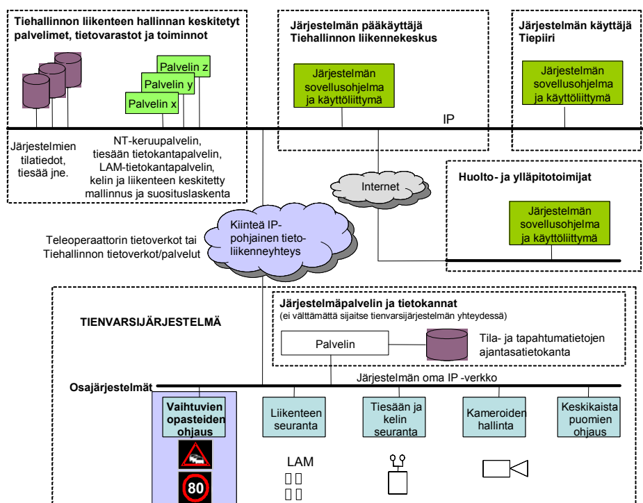
Kuva 24. Vaihtuvan ohjausjärjestelmän osat.
