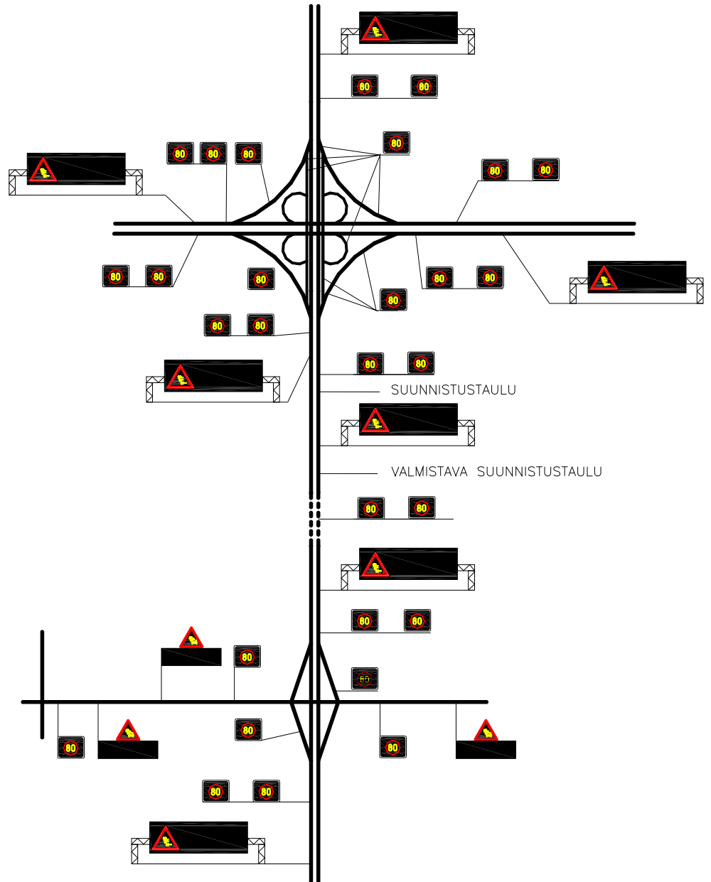
Kuva 20. Vaihtuvat opasteet nelikaistaisella keskikaistalla varustetulla tiejaksolla.
