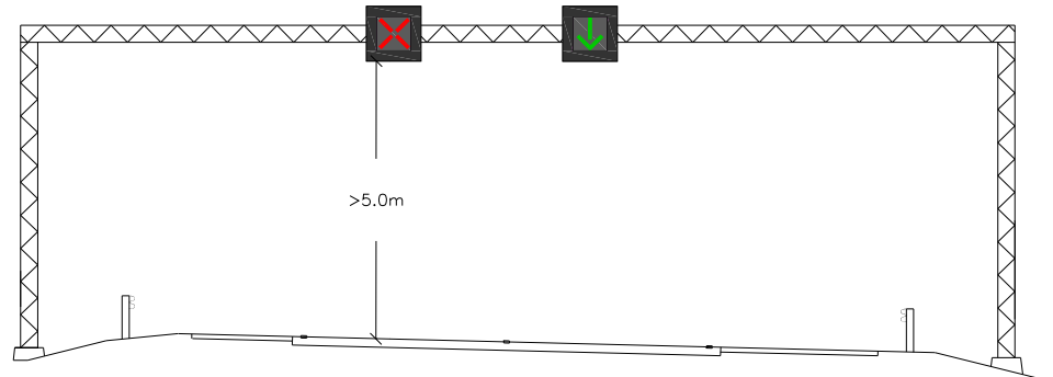
Kuva 17. Esimerkki kaistaopastimien sijoittamisesta nelikaistaisella keskikais- talla varustetulla tiellä. Kaiteen suojaetäisyys on huomioitava.
