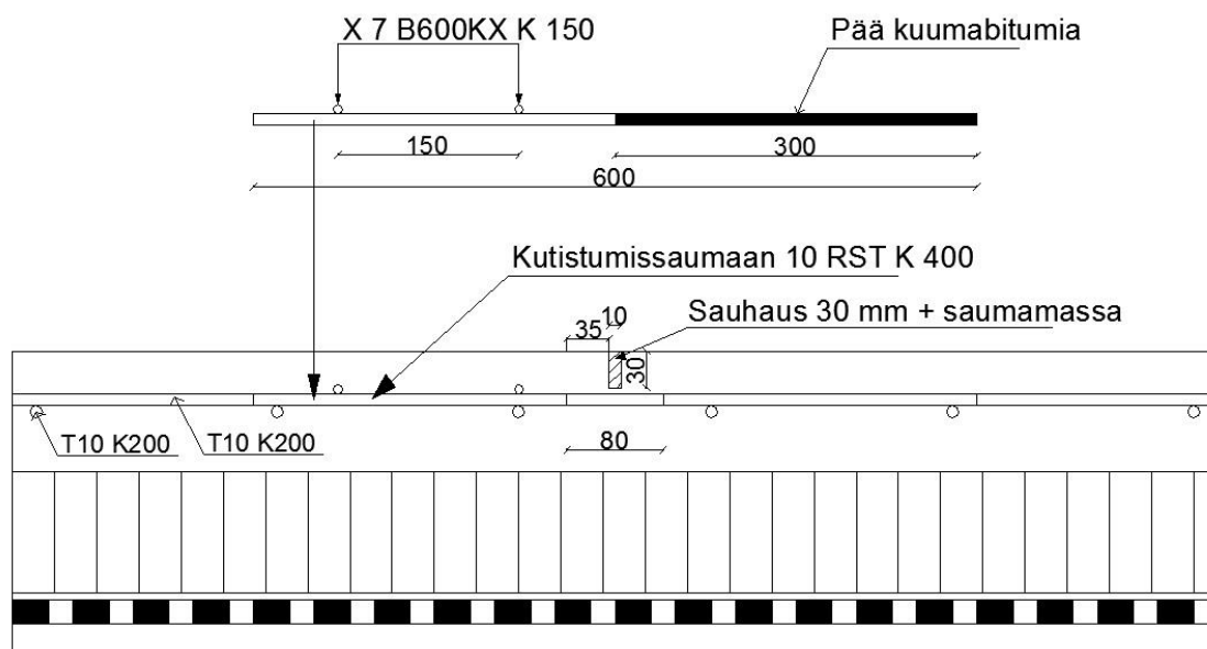
Kuva 17. Pystyleikkaus kutistumissauman kohdalta. Kuva Ville Väisänen
