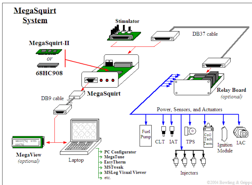
KUVA 11. Megasquirt-kaavio (13)
