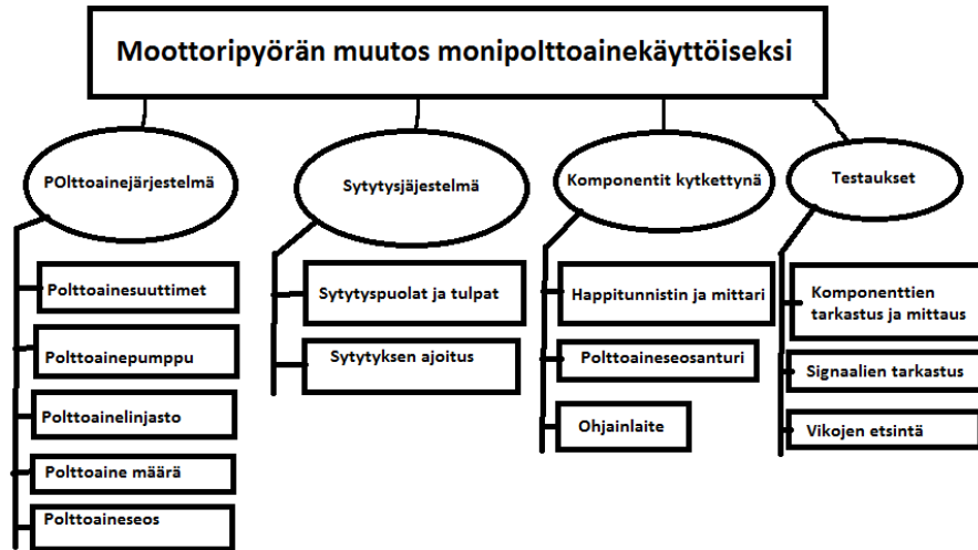
KUVA 22. Moottoripyörän muutos monipolttoainekäyttöiseksi
