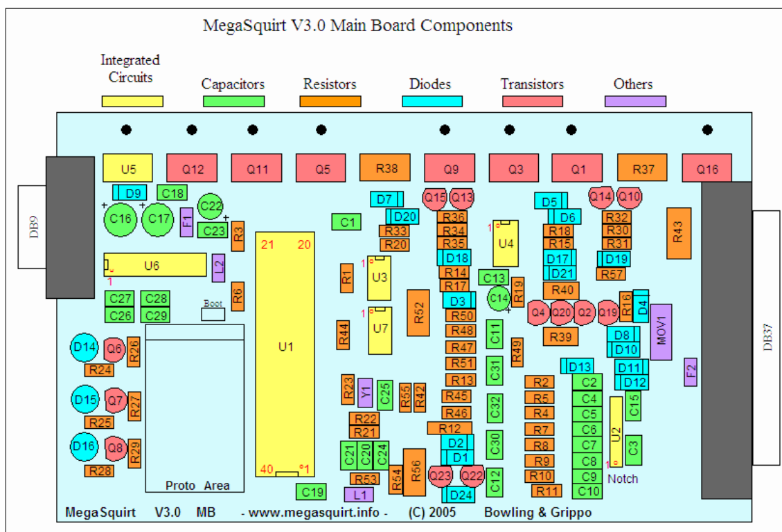
KUVA 13. Megasquirt-ohjainlaitteen komponenttikaavio (13)
