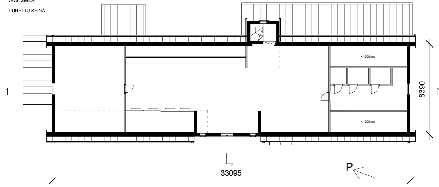
POHJAPIIRROS 2. KERROS 1:100
