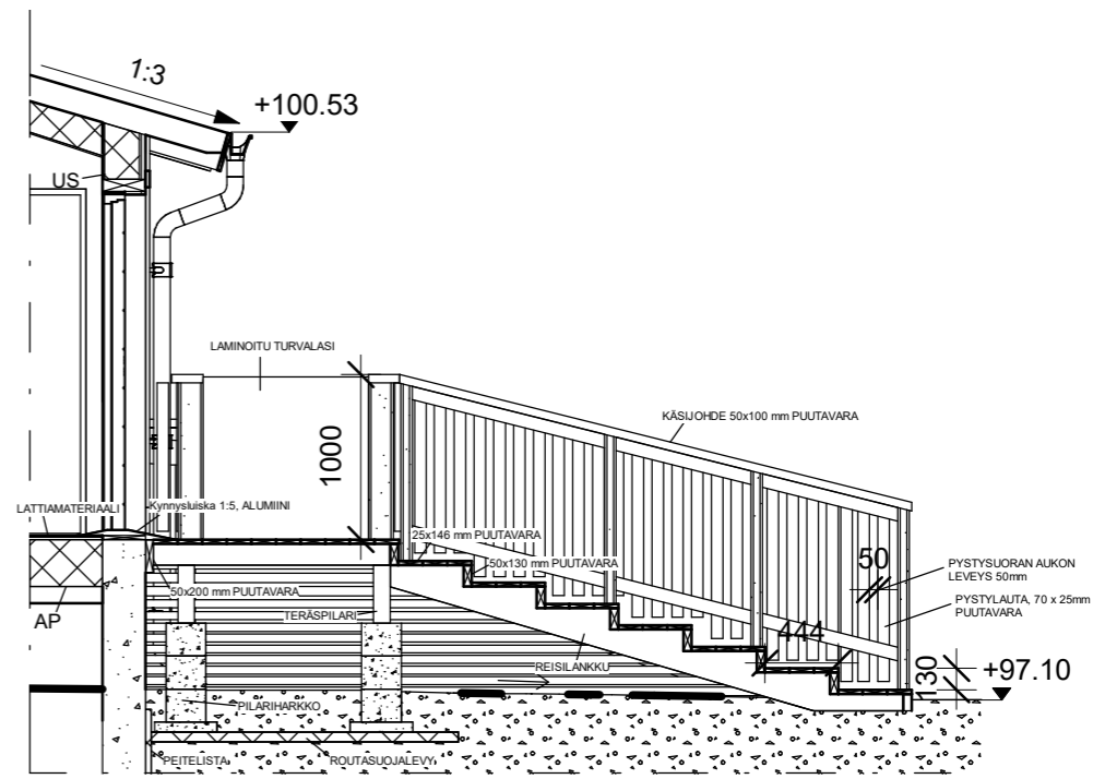
DETALJI- ULKOPORRAS 1:20
