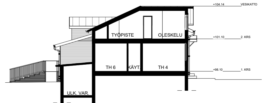
LEIKKAUS 1:100
