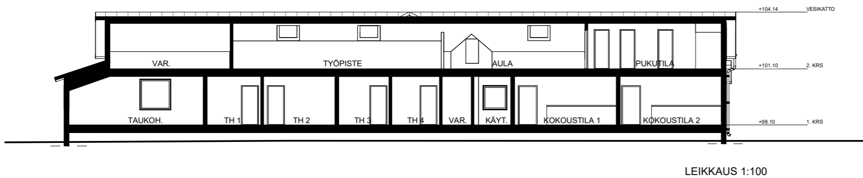
LEIKKAUS 1:100
