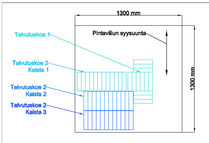
KUVIO 6. EN 310 -taivutuskokeeseen sahattujen koekappaleiden sijainti testivanerissa.
