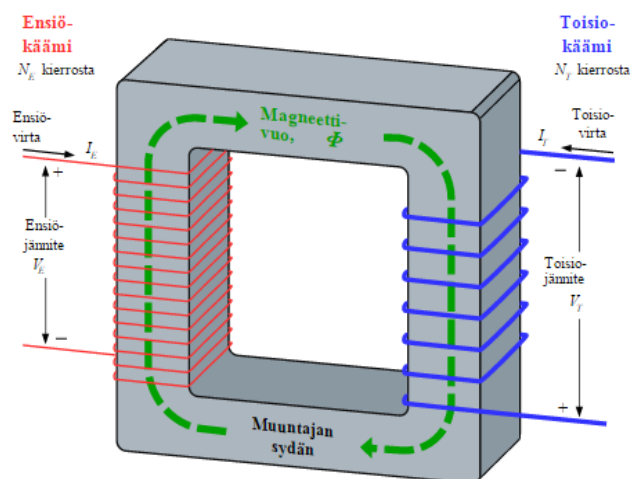
Kuva 12. Virtamuuntajan havainnekuva.
