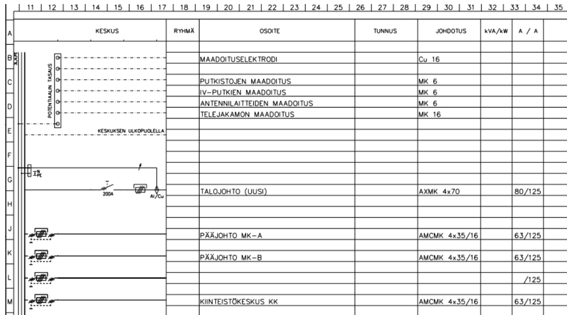
Kuva 4. Pääkeskuskaavio
