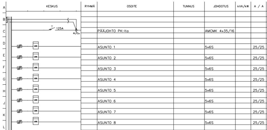
Kuva 5. Monimittauskeskuskaavio.
