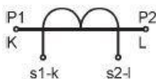
Kuva 13. Virtamuuntajan kytkentä. [13.]
